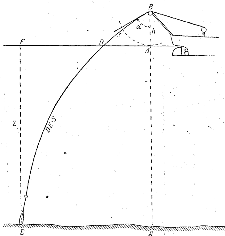
Рис. 7. Перемещение места нуля (М. О) при измерении глубин на ходу
