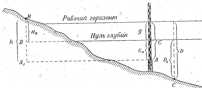
Рис. 20. Схема приведения измеренных глубин к нулю глубин.
