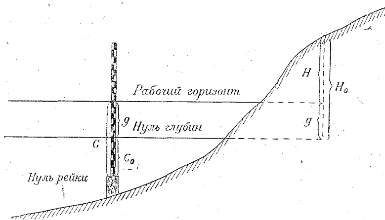
Рис. 4. Определение отметки береговой точки по высоте рабочего горизонта.
