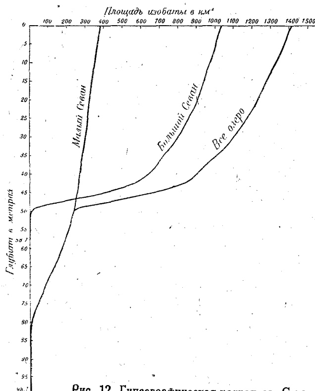
Рис. 12. Гипсографическая кривая оз. Севан.
