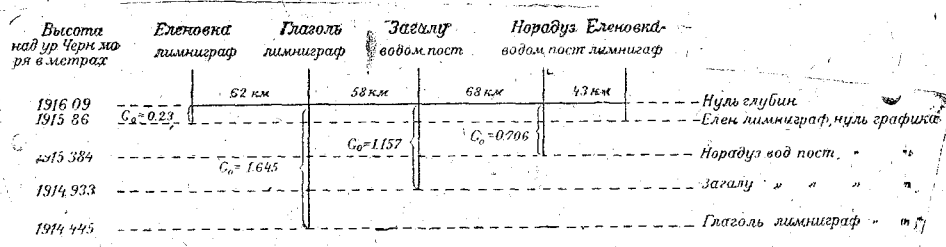
Рис. 3. Связь между нулем глубин Севанского Гидрометбюро и нулями графиков постоянной гидрометрической сети Бюро.
