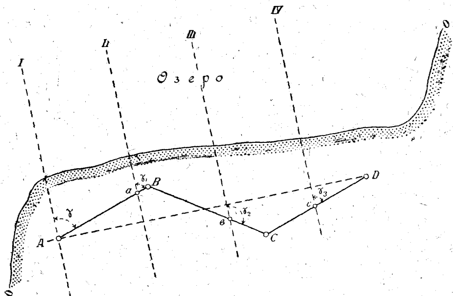
Рис. 14. Распланировка галсов шлюпочного промера по створам.
