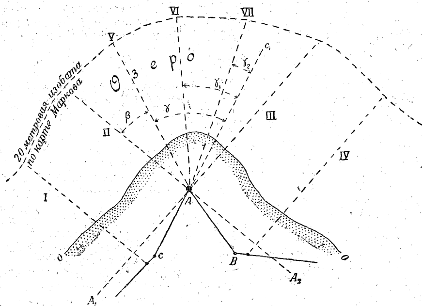
Рис. 15. Схема шлюпочного промера „звездочкой“.
