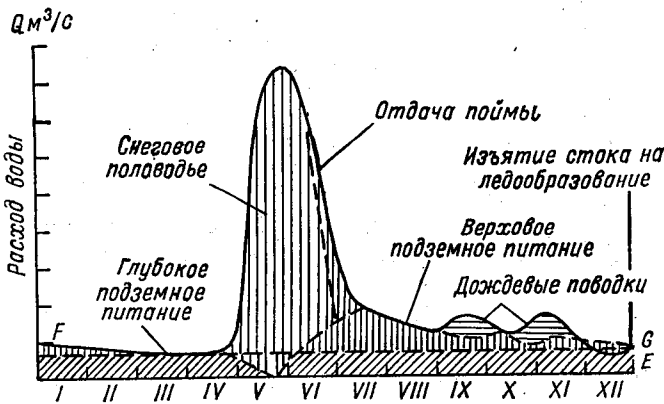
Рис. 6. Расчленение гидрографа р. Волги у г. Камышина.
