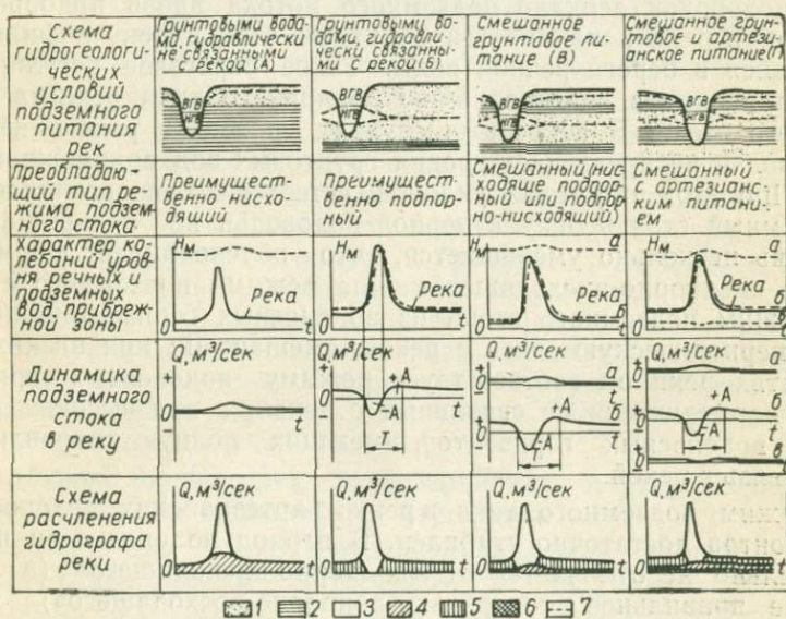
Рис. 1. Схемы гидравлической связи подземных и поверхностных вод (по Б. И. Куделину)
