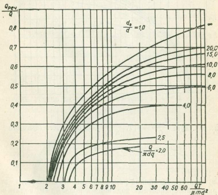
Рис. 15. График \frac{Q_{\text{реч}}}{Q} = f\left(\bar{T}, \frac{Q}{\pi d q}\right) для одиночного берегового водозабора при \beta = \frac{\pi}{2} и \frac{d_0}{d} = 1
