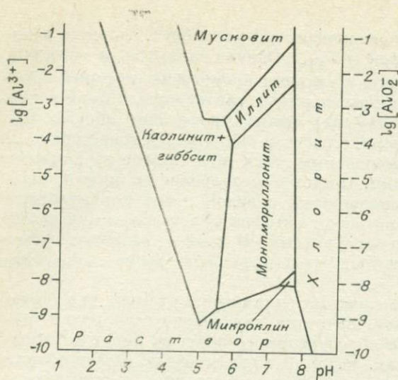
Рис. 4.2. Соотношения растворенных соединений алюминия с гипсбитом, каолинитом, иллитом и монтмориллонитом при различных значениях рН.
