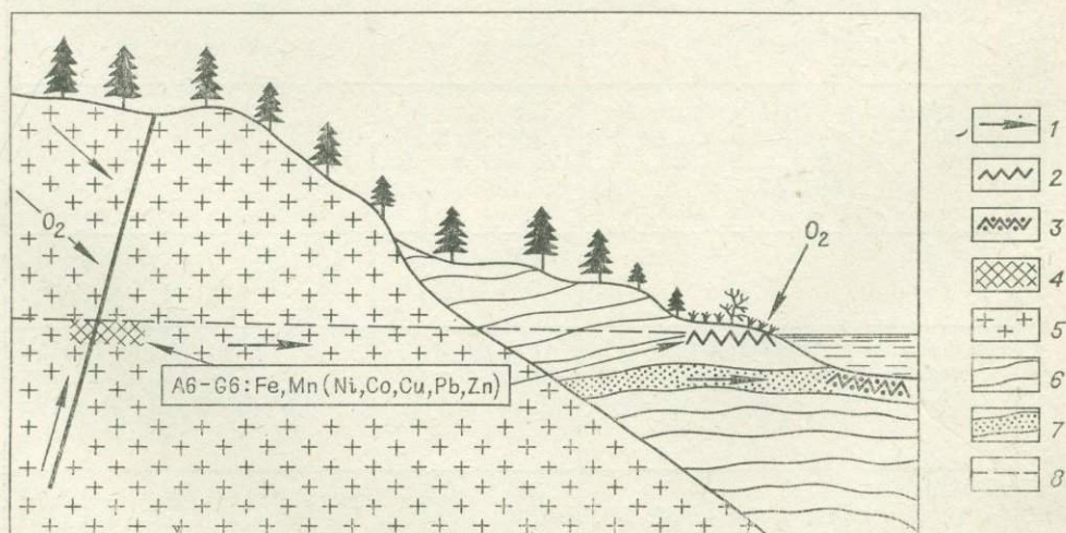
Рис. 5.6. Концентрации рудных элементов типа А6 — С6 на кислородном барьере зоны гипергенеза (по А. И. Перельману).
