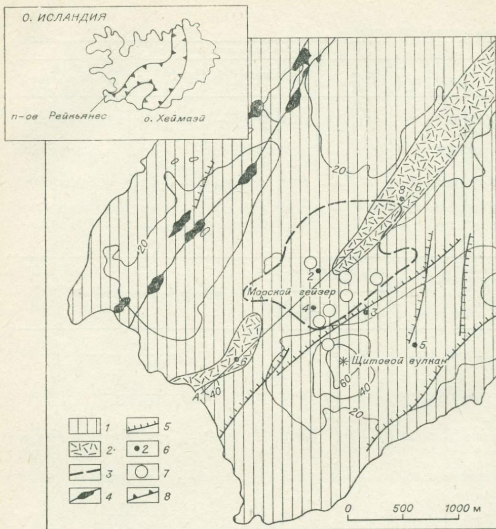
Рис. 8.1. Геологическая карта мыса Рейкьянес [Tomasson, Kristmannsdottir, 1972] 1 — постгляциальные базальтовые лавы щитовых вулканов и эруптивных трещин; 2 — палагоновые брекчии, туфы, пиллоу-лавы; 3 — граница месторождения термальных вод, проведенная по контуру зоны с \rho_K = 3 Ом·м [Björnsson e. a., 1972]; 4 — эруптивные трещины; 5 — сбросы; 6 — скважина и ее номер; 7 — термальные источники и фумаролы; 8 — граница Срединной неовулканической зоны.
