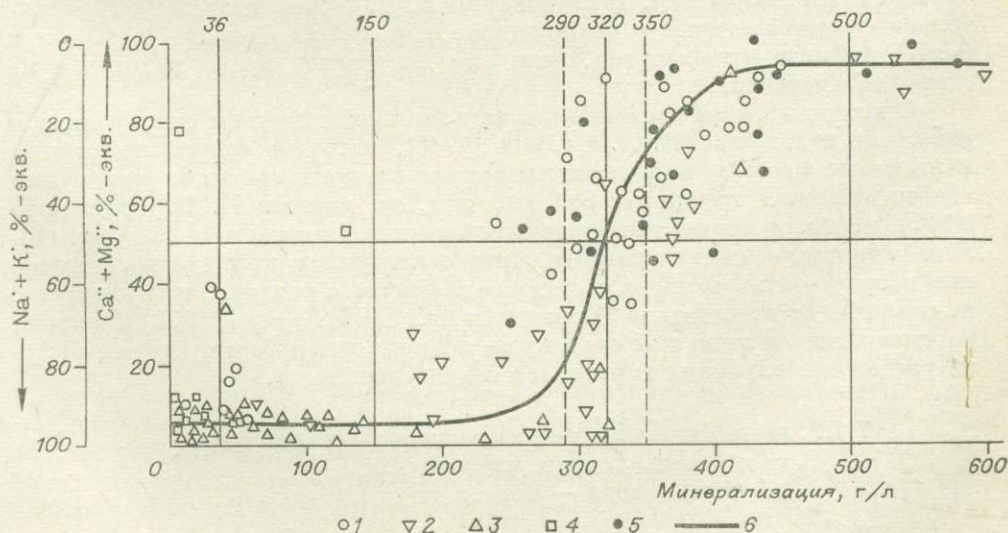
Рис. 7.8. Зависимость катионного состава от степени минерализации рассолов. Соленые воды и рассолы Ангаро-Ленского артезианского бассейна: 1 — терригенной формации 2 — соленосной формации, 3 — карбонатной формации, 4 — надсолевых отложений; 5 — рассолы из других регионов; 6 — линия средних значений.
