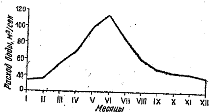
Схематическое распределение средних месячных расходов реки Каратал у станции Уш-Тобе.
