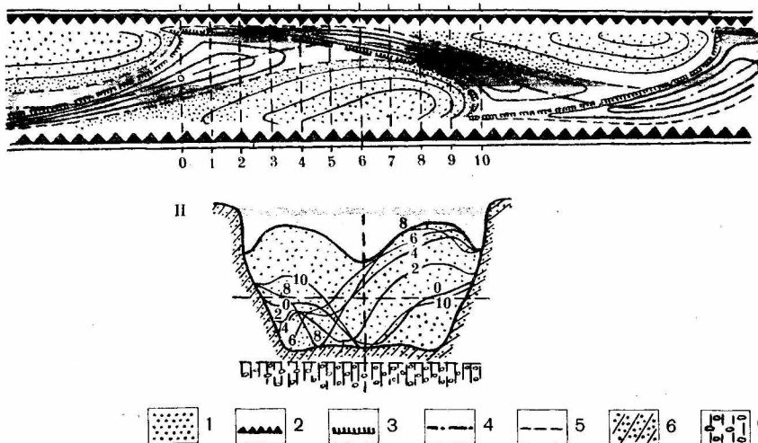
Схема графического определения отметок наибольшего размыва и намыва русла при ленточно-грядовом и побочном типах руслового процесса и при ограниченном меандрировании. План участка (I), совмещенные поперечные профили русла (II).
