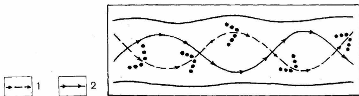
Рыбные ловушки древних индейцев, обнаруженные на аэрофотоснимках р. Потомак, по которым восстановлена линия старого фарватера реки.
