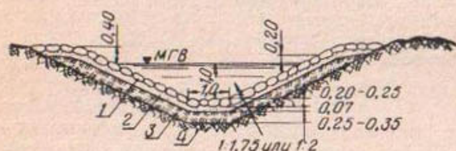
Рис. 37. Глиняная облицовка с защитным слоем из одиначной мостовой:
