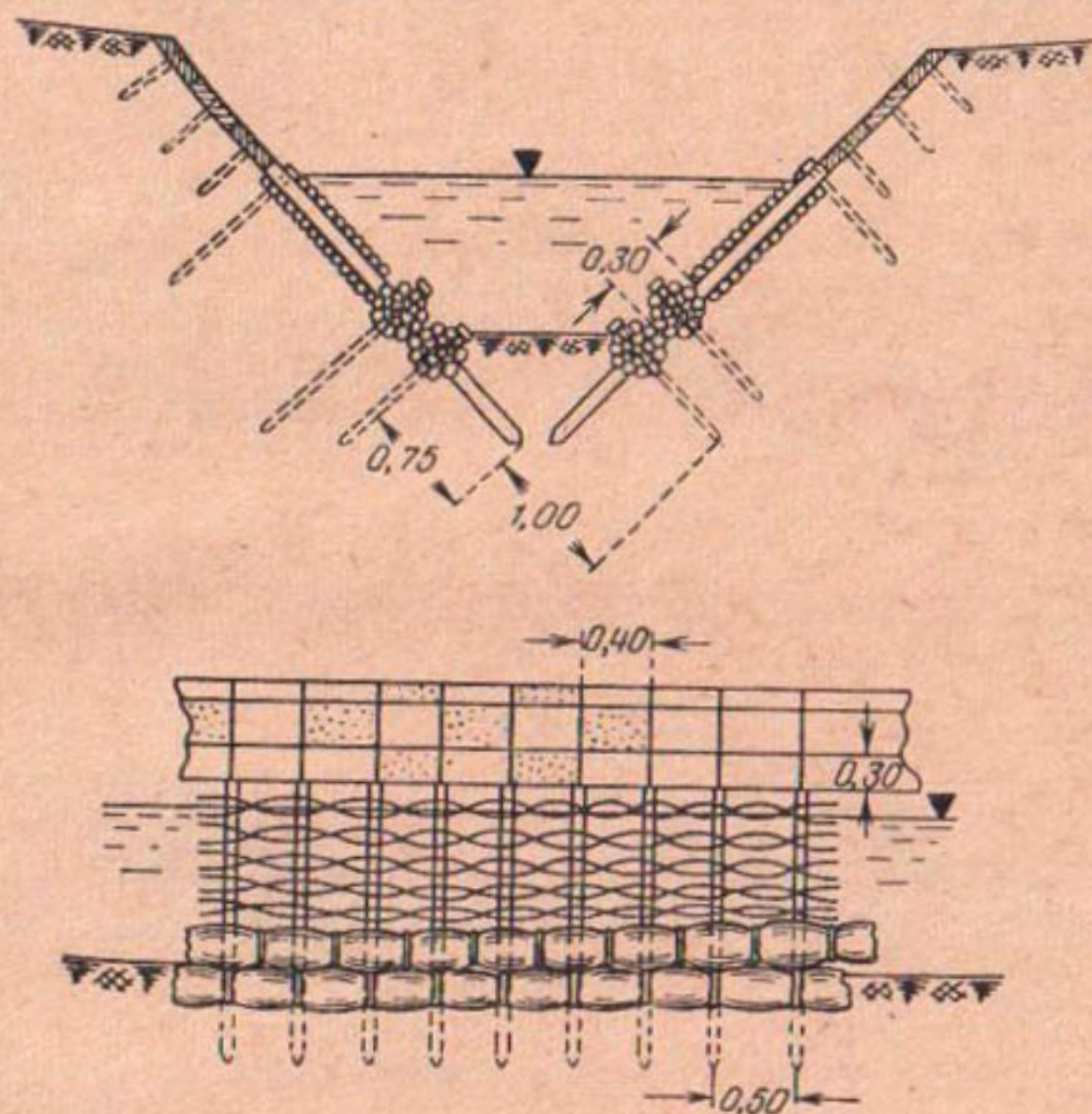
Рис. 53. Крепление откосов осушительного канала с применением фашины, плетня и дерна.
