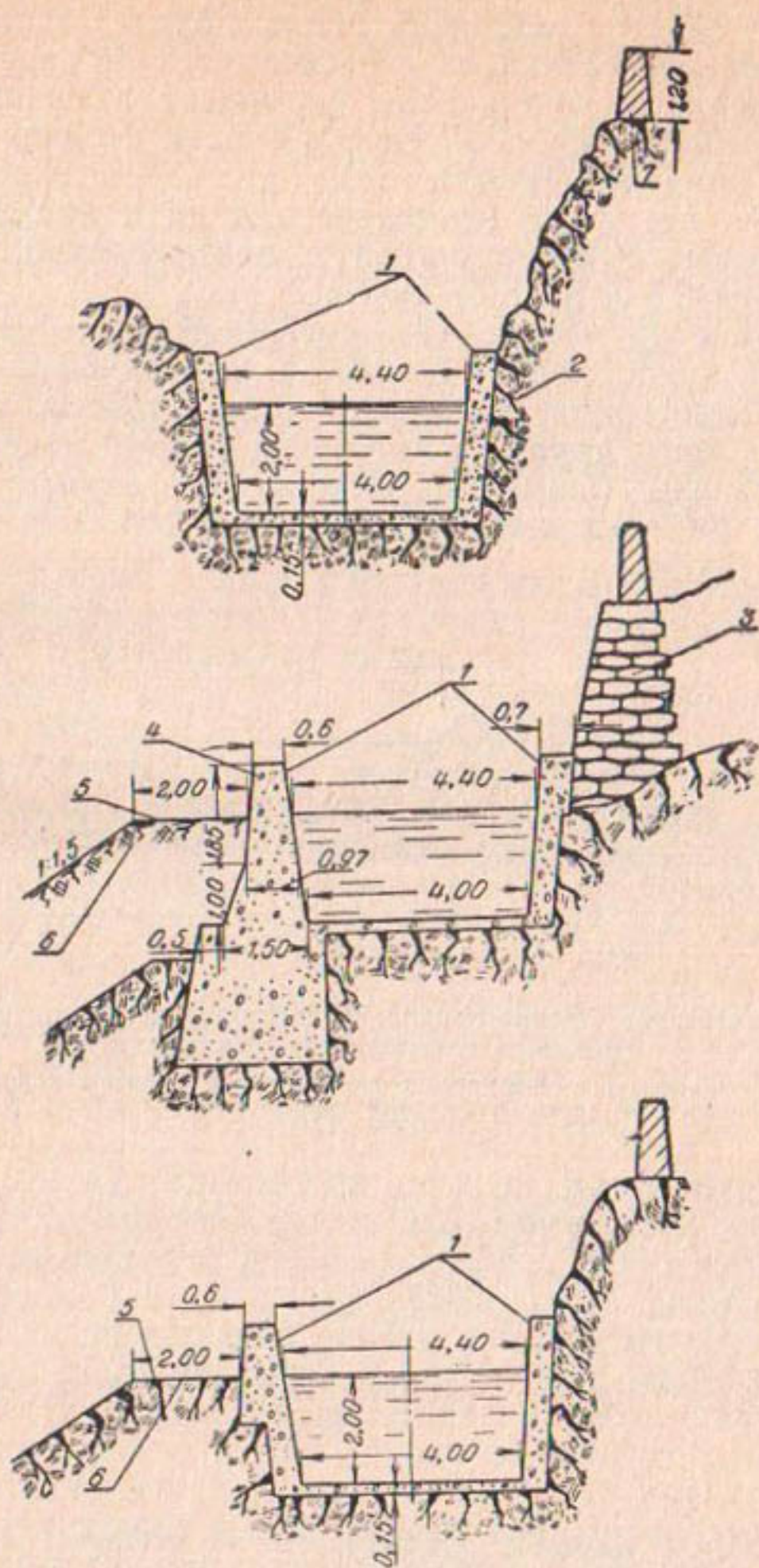
Рис. 12. Поперечные сечения канала на косогорных участках трассы:
