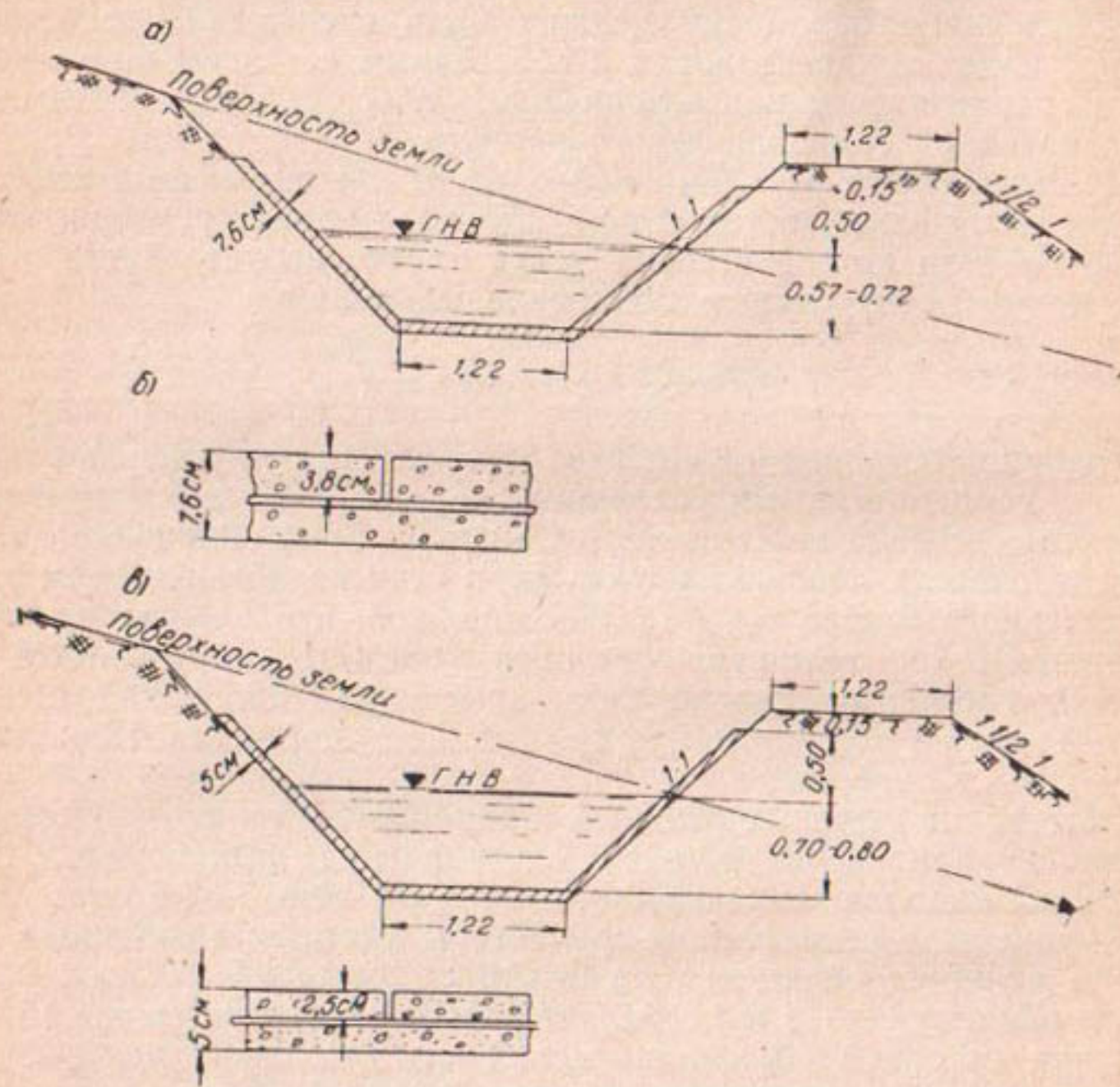
Рис. 25. Типовая конструкция бетонной (а) и торкретной (б) облицовок канала с деталями поперечных температурных швов (б и е).
