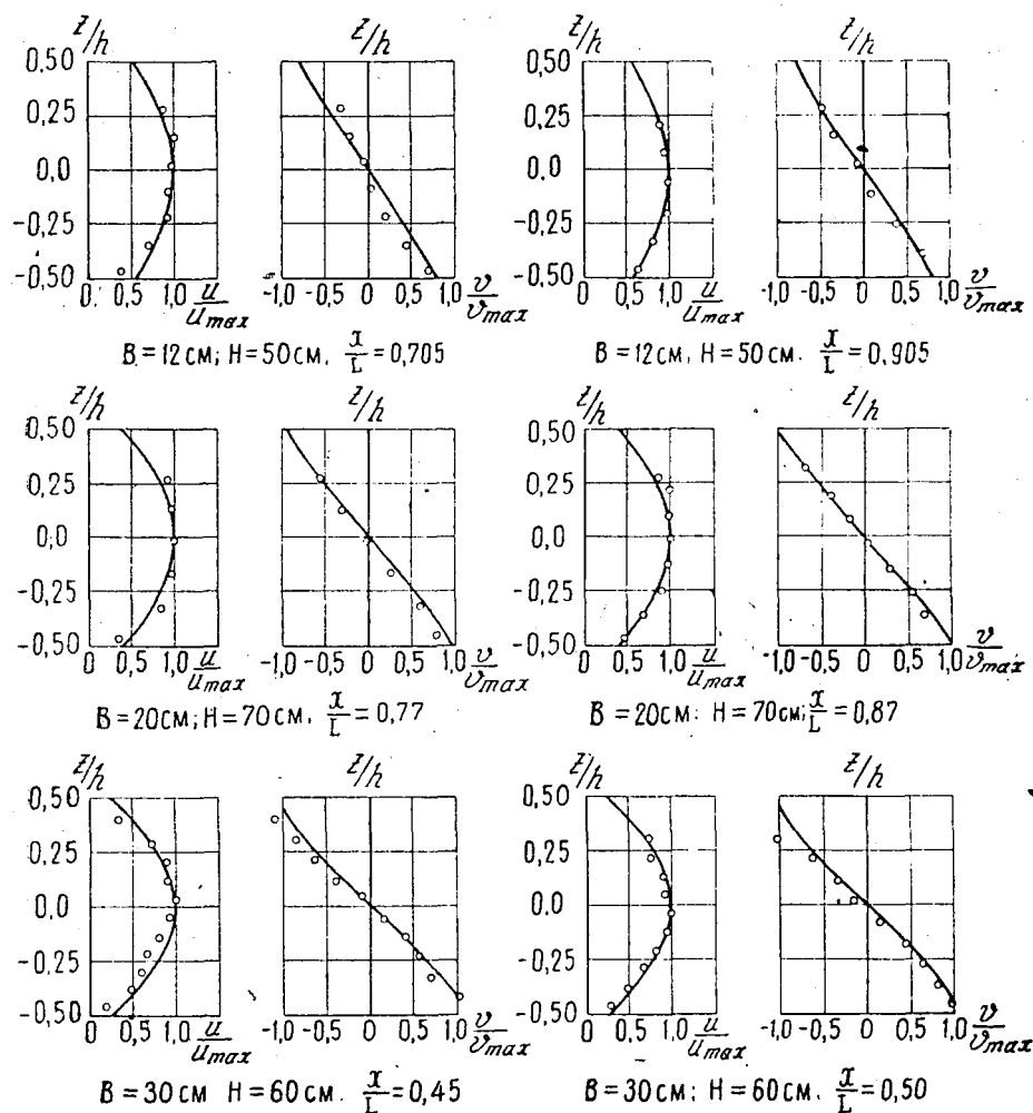
Рис. 3. Расчетные и опытные профили составляющих скорости в поперечных сечениях потока при различных величинах его ширины ( B ) и напорах ( H ).
