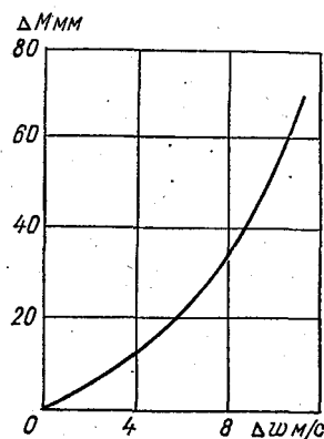
Рис. 4.6. Зависимость количества перенесенного ветром снега \Delta m_c от разности скоростей ветра при данном и предшествующем снегопаде \Delta w .
