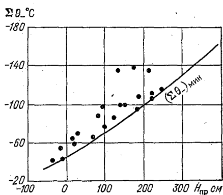
Рис. 2.1. Зависимость суммы средних суточных отрицательных значений температуры воздуха \Sigma\Theta_{-} за период от появления льда до начала ледостава от уровня воды H_{пр} в день, предшествующий началу ледостава.
