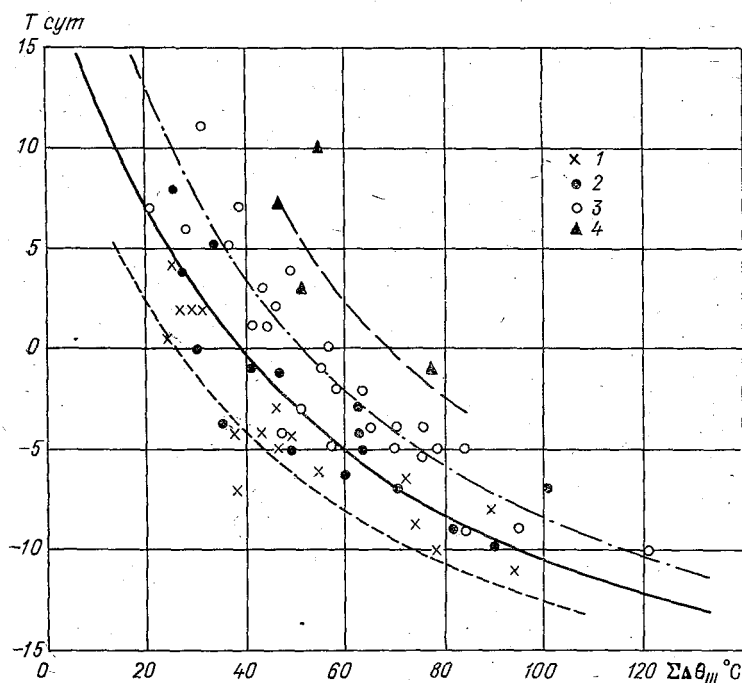
Рис. 8.3. Зависимость отклонения от нормы сроков вскрытия рек бассейна Верхней Оби T от суммы потеплений в марте \sum \Delta\theta_{\text{III}} с учетом высоты снежного покрова в Северном Казахстане и на Алтае и аномалии давления в марте.
