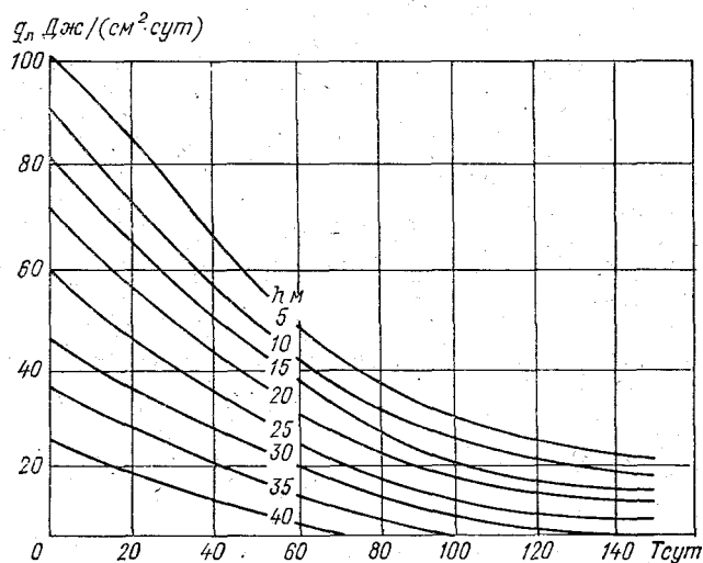
Рис. 4.4. Зависимость суточного притока тепла от грунта q_n от продолжительности ледоставного периода T и средней глубины водоема h .
