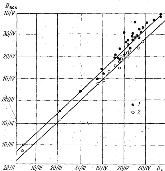
Рис. 7.2. Обобщенная связь даты начала дрейфа льда (вскрытия) с датой накопления суммы тепла, необходимой для таяния льда толщиной ( h_{\text{макс}} = 15 см).
