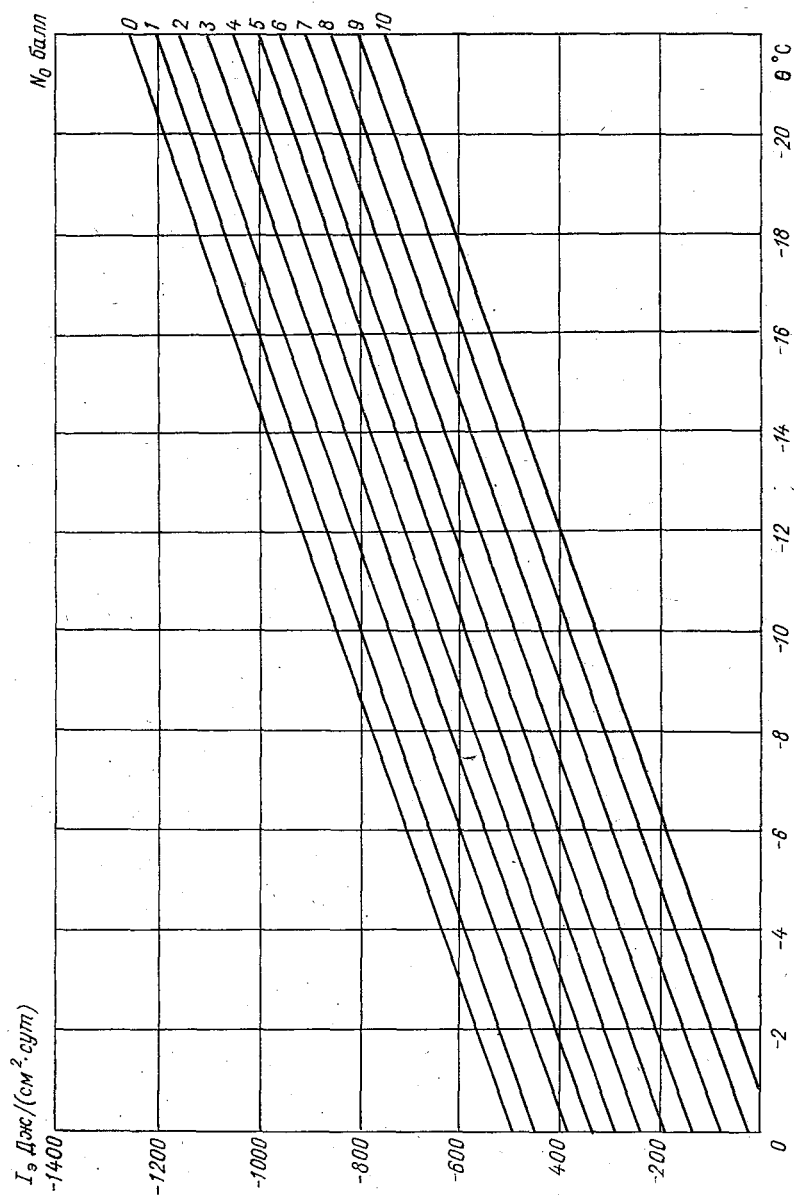
Рис. 1.4. Номограмма для определения эффективного излучения I_0 при температуре поверхности воды \theta \text{ } ^\circ\text{C} .
