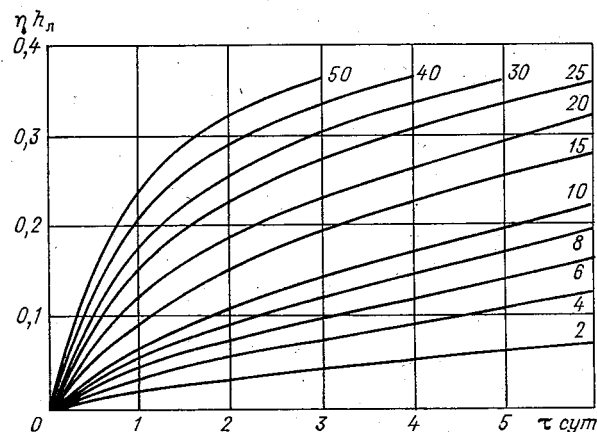
Рис. 1.7. Номограмма для расчета произведения \eta h_{\text{л}} . Цифры у линий — теплообмен водной поверхности, \text{Дж}/(\text{см}^2 \times \text{сут}) .
