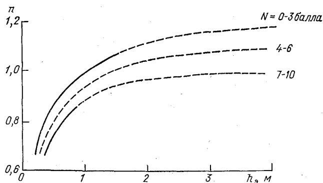
Рис. 4.3. Зависимость соотношений температур поверхности снежно-ледяного покрова \vartheta_{пл} и воздуха \Theta при большой толщине льда от эквивалентной толщины льда h_э и облачности N .
