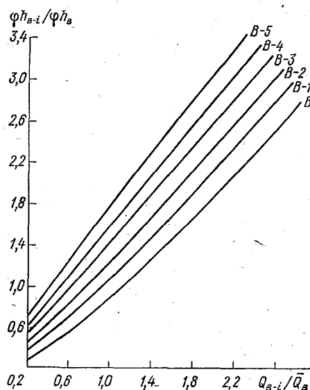
Рис. 6.5. Связь модульных коэффициентов прочности льда и расходов воды за дни, предшествующие вскрытию ( в - i ).
