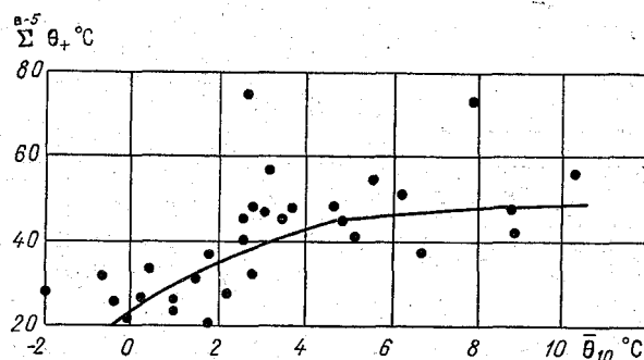
Рис. 6.8. Зависимость суммы средних суточных положительных значений температуры воздуха (без температуры за 5 сут до вскрытия), необходимой для вскрытия
