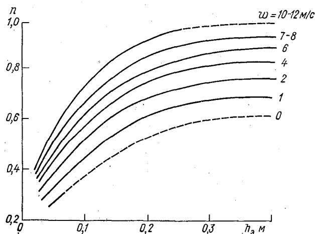
Рис. 4.2. Зависимость соотношений температур поверхности снежно-ледяного покрова и воздуха n = \frac{\vartheta_{пл}}{\Theta} при малой толщине льда от эквивалентной толщины льда h_э и скорости ветра \omega .
