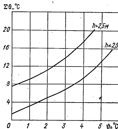
Рис. 1.5. Зависимость суммы средних суточных отрицательных значений температуры воздуха \sum \Theta_- , необходимой для появления льда, от начальной температуры воды \vartheta_0 и средней глубины h на р. Северная Двина у Абрамкова.
