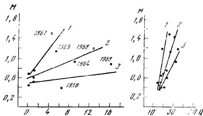
Рис. 15. Зависимость минерализации ( M , г/л) в бассейне Кашкадарьи: А — от русловой приточности ( Q_{\text{рус. прит.}} , м³/с); Б — водозабора ( Q_{\text{вб.}} , м³/с)
