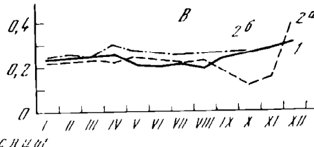
Рис. 11. Хронографы минерализации 1938 г. в водах рек
