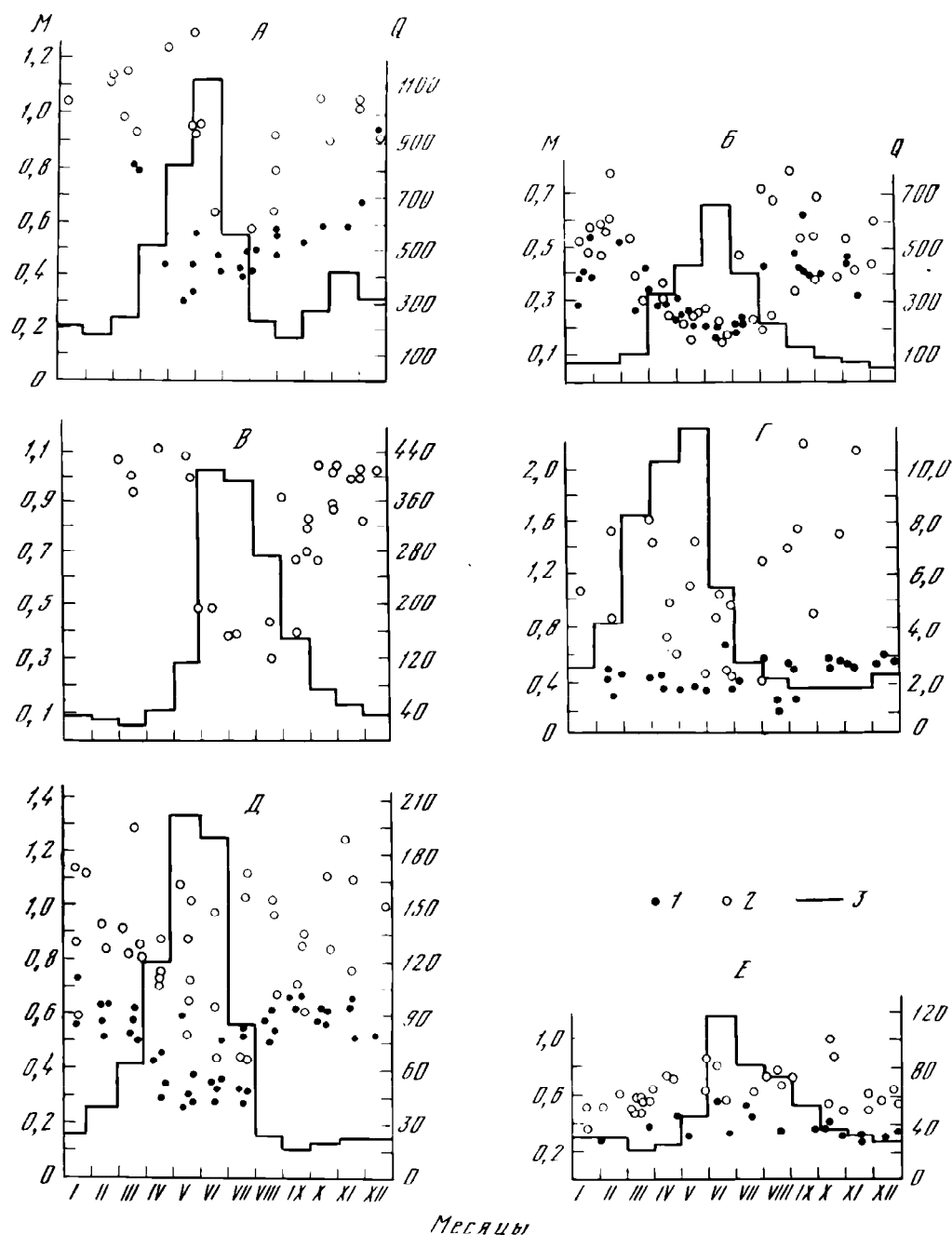
Рис. 12. Общее увеличение минерализации ( M , г/л) в замыкающих створах рек за многолетний период при различных расходах воды ( Q , м³/с)
