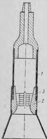
Рис. 86. Шлипс: 1 — корпус шлица; 2 — конус; 3 — плашки.
