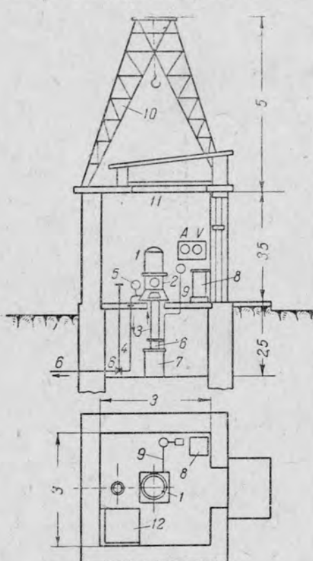
Рис. 38. Павильон для установки вертикального центробежного насоса:
