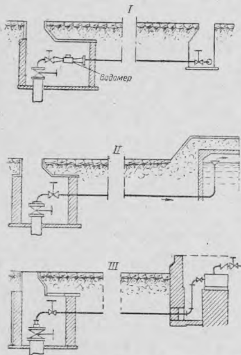
Рис. 30. Подача воды из самоизливающихся скважин:
