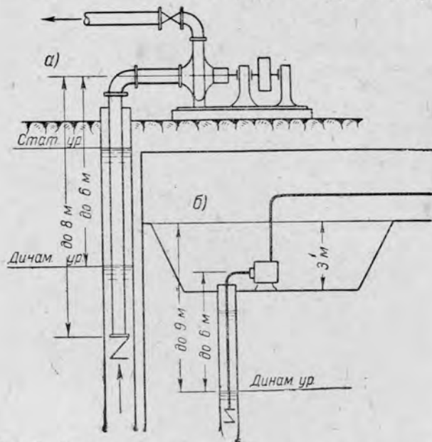
Рис. 5. Определение дебита скважин при динамическом уровне до 9 м ниже поверхности земли: а — насос установлен на поверхности земли; б — насос установлен в выемке.
