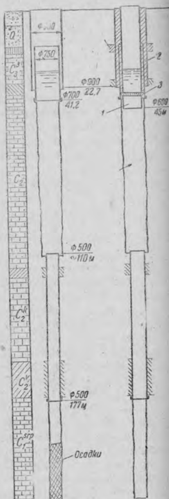
Рис. 76. Пример восстановления скважины закреплением клепаными обсадными трубами:
