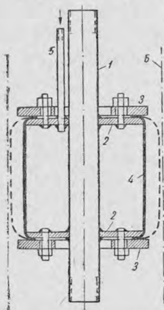
Рис. 63. Пневматическая пробка:
