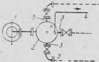
Рис. 33. Подача воды из скважины несколькими насосами:
