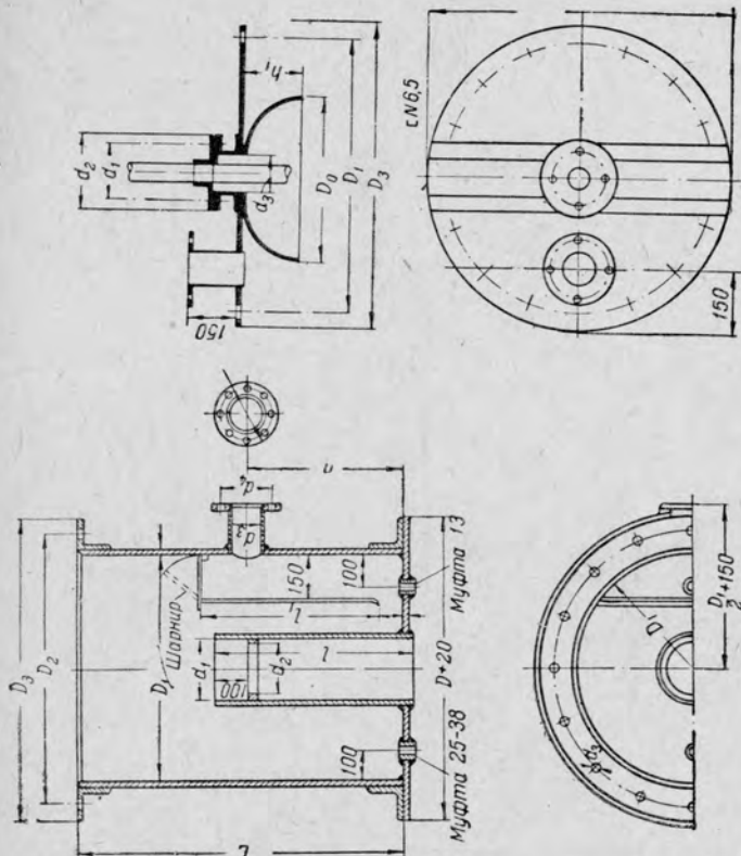
Рис. 56. Приемный бак.
