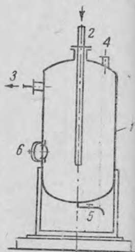
Рис. 49. Ресивер: 1 — ресивер; 2 — воздушная труба от компрессора; 3 — труба на ресивера к шлиту управления; 4 — штуцер для предохранительного клапана; 5 — отверстие для спуска конденсата; 6 — люк.
