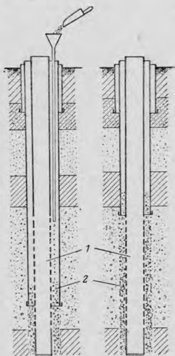
Рис. 26. Обсадной гравийный фильтр:
