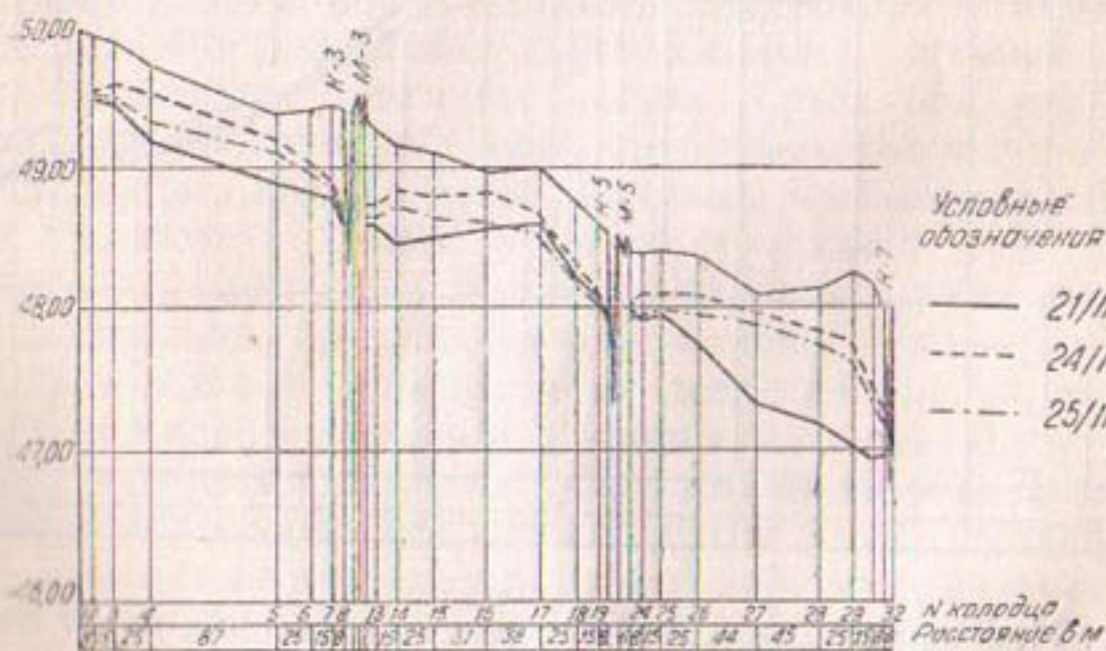
Рис. 10. Влияние дождя на уровень грунтовых вод.
