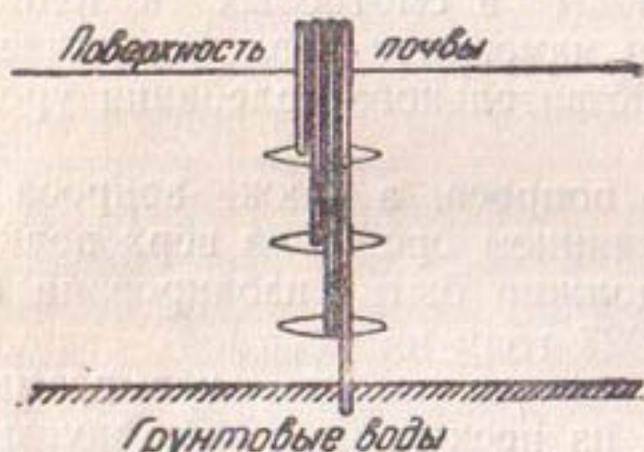
Рис. 1. Сложный колодец.
