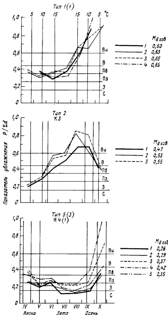
Рис. 5. Типы атмосферного увлажнения сельскохозяйственных сезонов по агро-Увлажнение сельскохозяйственных сезонов: Ви — избыточно влажно, В — влажно, Пв — по-Тарту, 3 — Петрозаводск, 4 — Киров; тиг 2: 1 — Хабаровск, 2 — Бикин, 3 — Завитинск; 6(2): 1 — Новоселенгинск, 2 — Улан-Удэ, 3 — Агинское, 4 — Чита, 5 — Шимановск, 6 — Благо-12(1): 1 — Ташауз, 2 — Ербет,
