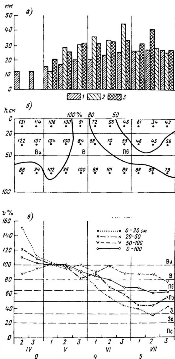
Рис. 13. Влагообеспеченность по запасам почвенной влаги. Провинция IV-3, ст. Немчиновка, Московская обл., яровые культуры. Усл. обозначения см. рис. 12.
