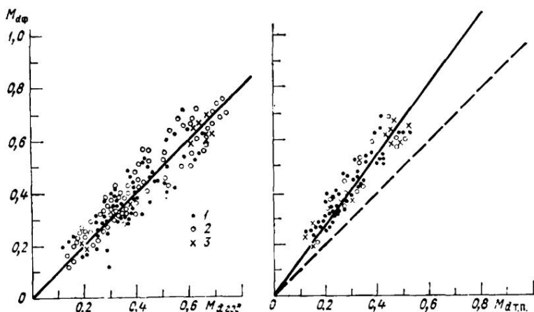
Рис. 3. Соотношение показателей увлажнения, вычисленных по фактическому испарению M_{дф} и по осадкам теплого периода M_{дт.п.} .
