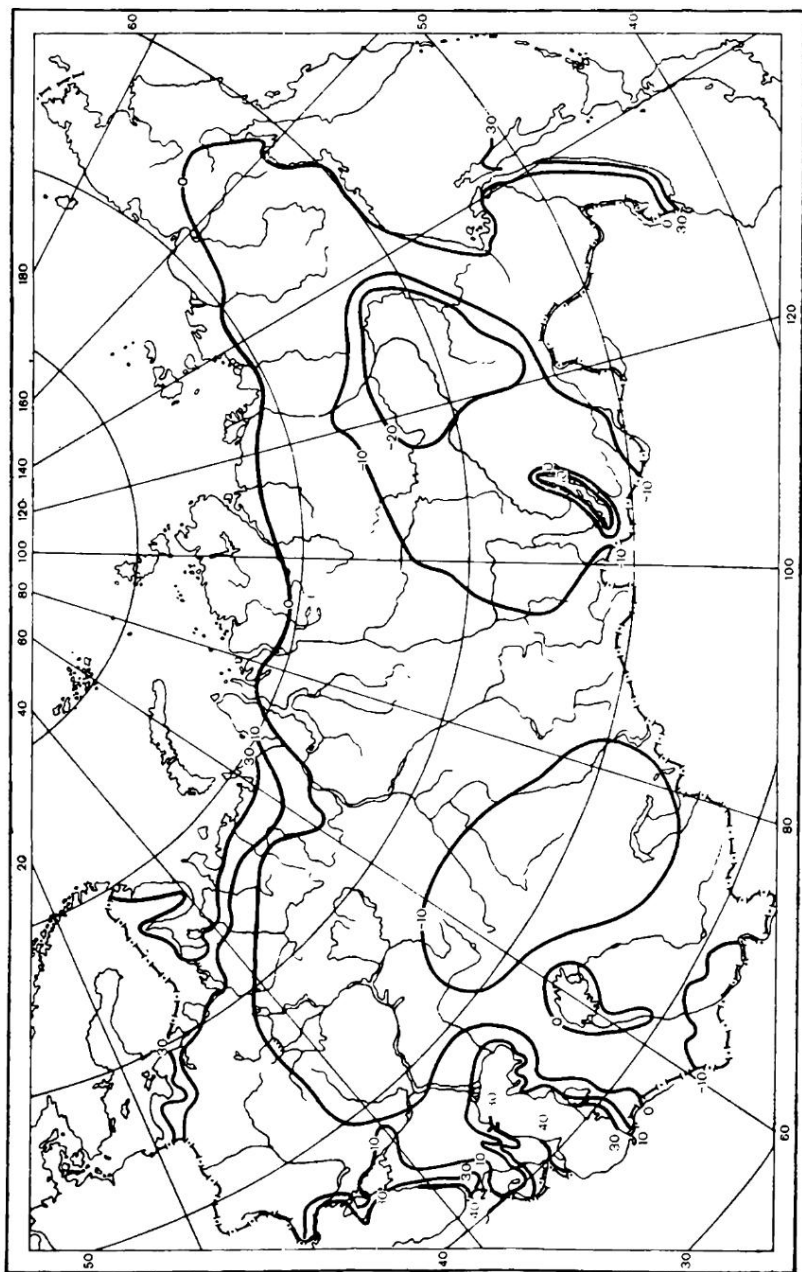
Рис. 11. Отклонение (дни) беззаморозкового периода от основного.
