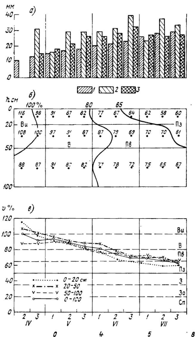
Рис. 12. Влагообеспеченность по запасам почвенной влаги. Провинция IV-1, ст. Каунас, Литовская ССР, яровые культуры.
