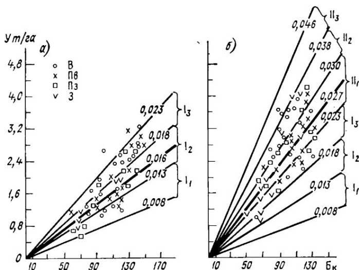
Рис. 23. Связь урожайности зерновых культур при разных уровнях интенсивности земледелия со значениями биоклиматического потенциала ( B_k = 55 БКП). а — в хозяйствах, б — на госсортоучастках. Зоны увлажнения: В — влажная лесная, Пв — полувлажная лесостепная, Пз — полусухая степная, З — засушливая степная и сухостепная. Римские цифры с индексом — уровни биологической продуктивности (см. табл. 57).
