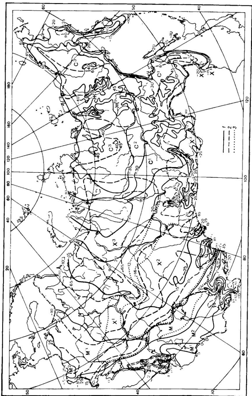
Рис. 8. Суровость и снежность зимы (подробную легенду см. в табл. 18, 19). 1 — температура воздуха наиболее холодного месяца, °C; 2 — высота снежного покрова, см; 3 — средняя температура воздуха на глубине узла кушения, °C.
