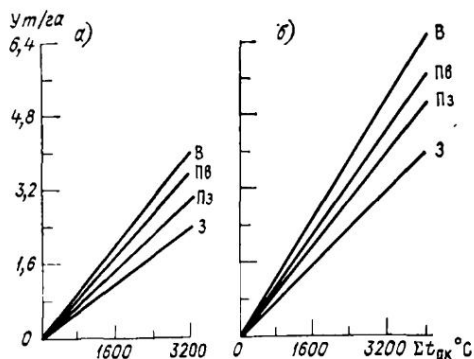
Рис. 18. Связь урожайности озимой пшеницы (а) и кукурузы (б) с теплообеспеченностью ( \Sigma t_{ак} ) по зонам увлажнения.
