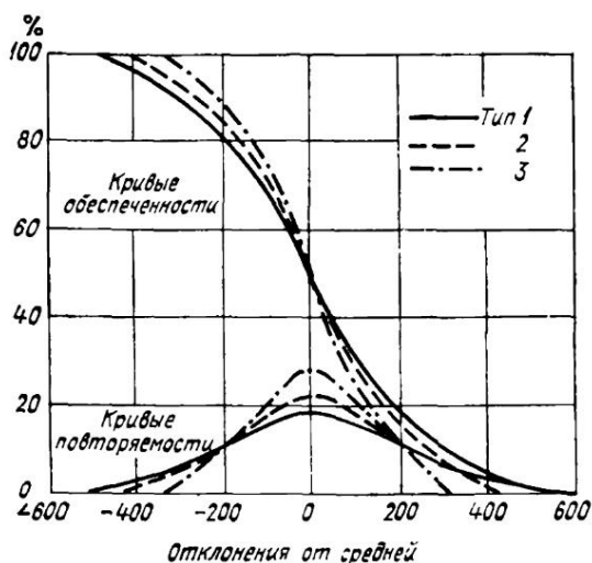
Рис. 1. Кривые обеспеченности и повторяемости сумм температур за период с температурой выше 10 °C.
