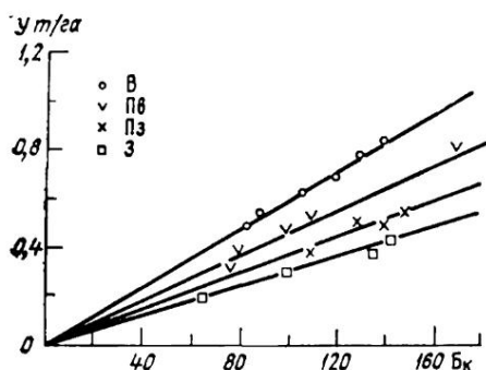
Рис. 25. Связь прироста урожайности зерновых культур по НРК со значениями климатического индекса биологической продуктивности B_k .
