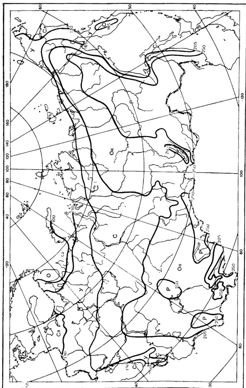
Рис. 9. Континентальность климата СССР (по Н. Н. Иванову). О — океанический ( K < 100 ); Сл — слабоконтинентальный ( K = 100 \dots 130 ); У — умеренно континентальный ( K = 130 \dots 165 ); С — среднеконтинентальный ( K = 165 \dots 205 ); Ок — очень континентальный ( K = 205 \dots 250 ); Р — резко континентальный ( K > 250 ).
