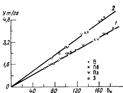
Рис. 22. Связь урожайности ( Y ) со значениями климатического индекса биологической продуктивности ( B_k ). 1 — озимая пшеница, 2 — кукуруза. Зоны увлажнения см. рис. 18.
