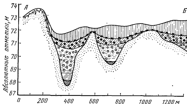
Рис. 3.7. Разрез А—Б местности (см. рис. 3.2) с разными видами торфа (см. рис. 2.9) [3.2]. На вертикальной оси указана высота над нормальным нулем.
