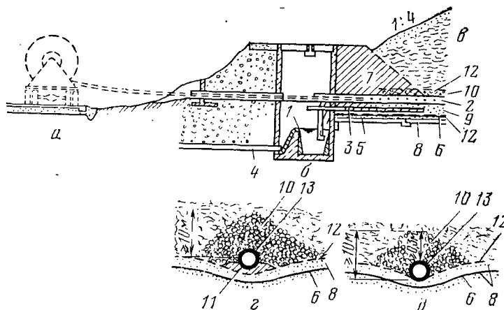
Рис. 7.25. Дренаж с контрольной шахтой для обычного отвала мусора (высота отсыпки до 30 м) и для большого отвала с высокой отсыпки до 100 м [7.34]:
