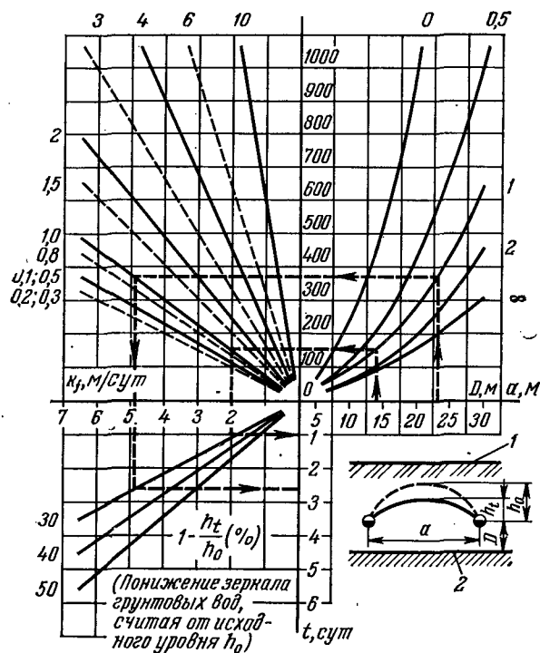
Рис. 6.16. Номограмма для определения продолжительности осушения [6.2]:
