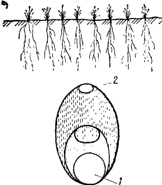
Рис. 5.15. Изменение сечения кротовой дрены вследствие переотложения почвы [4.6]:
