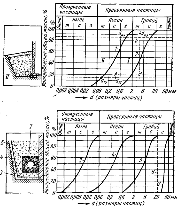
Рис. 7.14. Правила устройства фильтров Терцаги (стандарт ФРГ DIN 4095):
