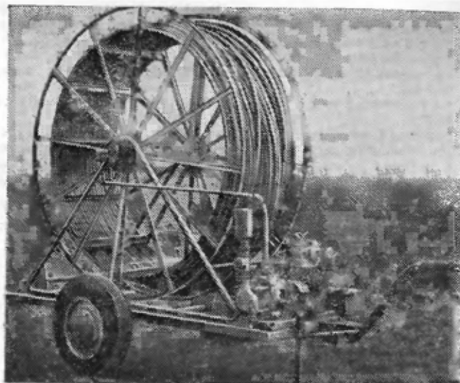
Рис. 10.3. Дренопромывочный аппарат типа «Диема».
