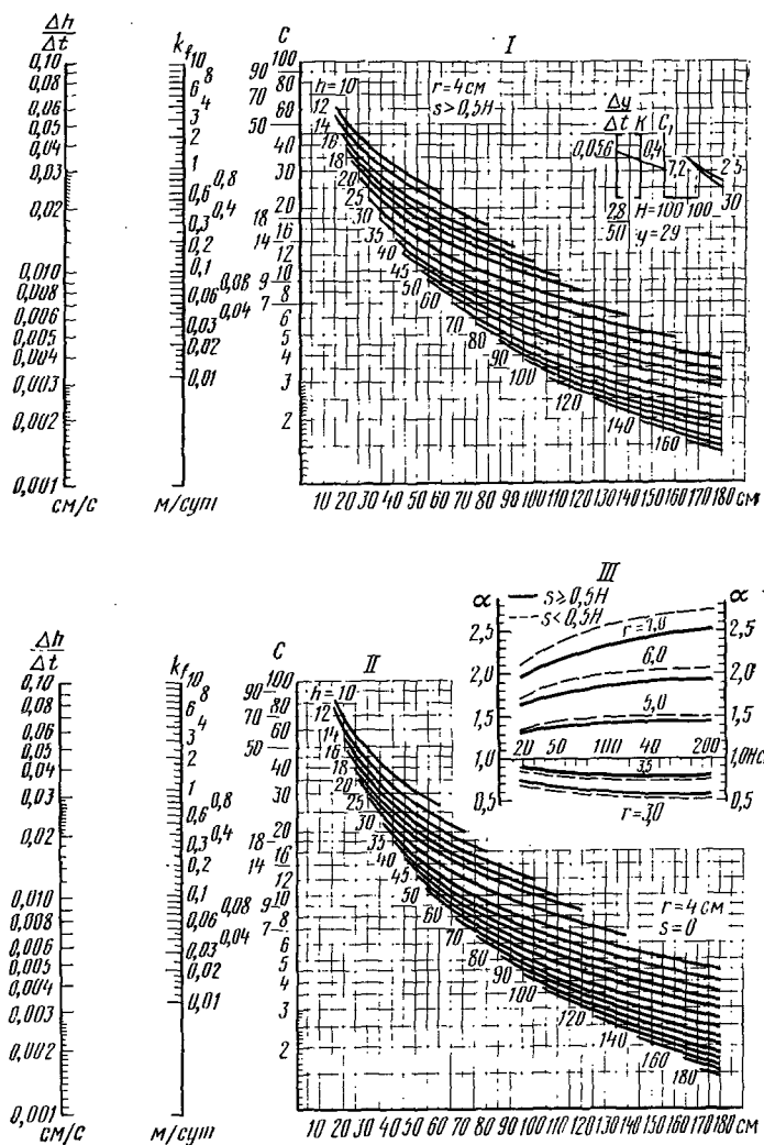
Рис. 3.13. Номограммы для определения в полевых условиях фильтрационной способности k_f при r=4 см [3.3]: I — для s \geq 0.5H ; II — для s < 0.5H ; III — для радиуса скважин r \neq 4 см.
