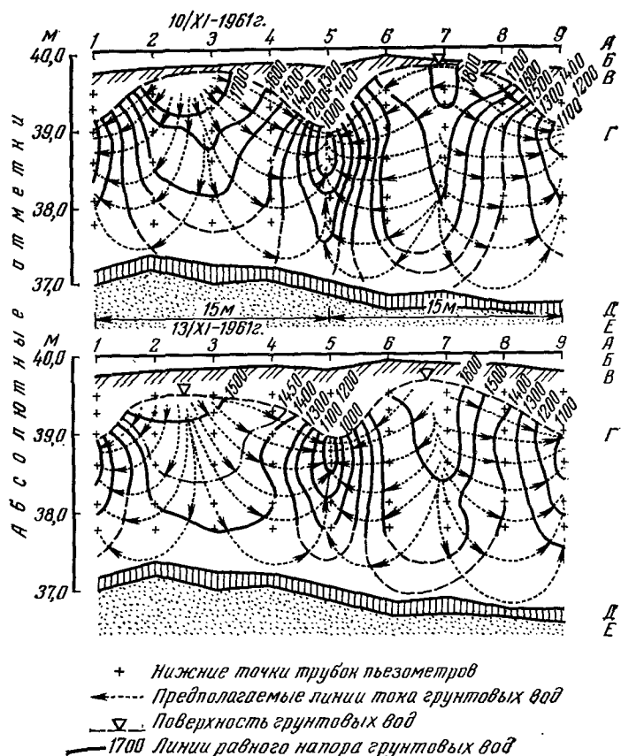
Рис. 5.3. Линии равного напора грунтовых вод и линии тока, полученные в результате пьезометрических измерений между трубчатыми дренами:
