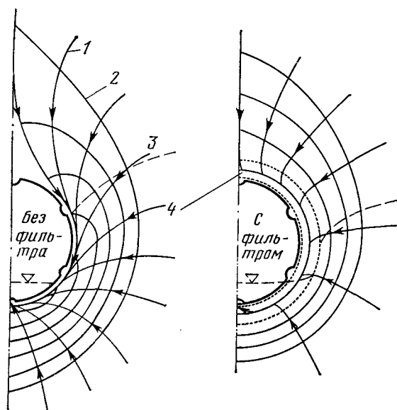
Рис. 5.13. Линии равного напора и линии тока воды при частичном заполнении дренажной трубы с дренажным фильтром и без него [5.7]:
