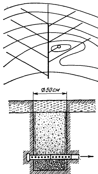
Рис. 7.8. Осушение поверхностных мульд шлюккерами и дополнительными коллекторами [7.10].
