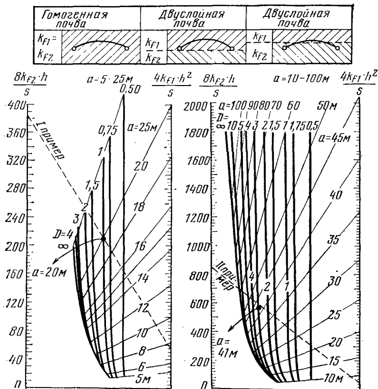
Рис. 6.7. Номограмма для определения расстояний между дренами на почвах, заболоченных грунтовыми водами [6.1].
