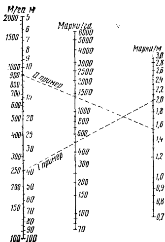
Рис. 4.10. Номограмма для определения общей протяженности дрен и затрат на их строительство.
