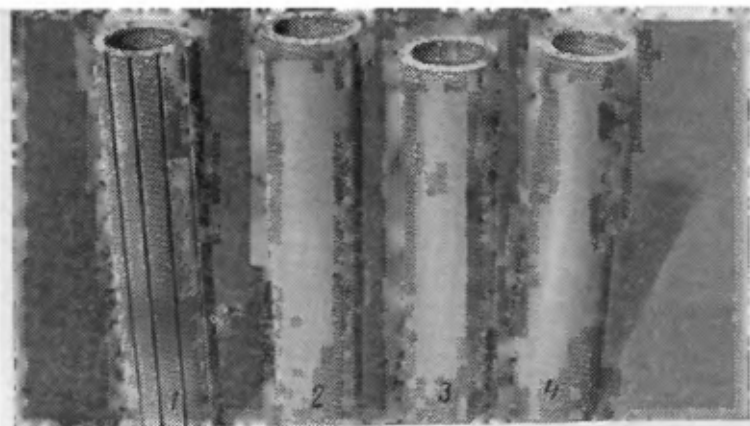
Рис. 8.4. Гончарные трубы:
