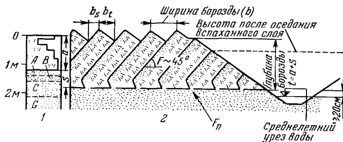
Рис. 4.9. Схема естественного профиля почвы на верховом болоте и профиля после глубокой вспашки при необходимой глубине осушения:
