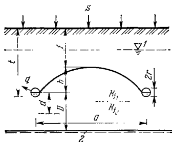
Рис. 6.6. Схема к формуле расчета расстояний между дренами [6.1]:
