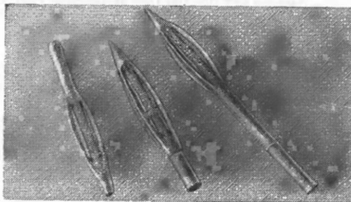
Рис. 10.1. Струйчатые трубы аппарата для промывки дрен: Слева направо: вперед, назад, в сторону [10.2].
