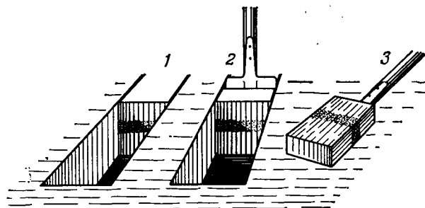
Рис. 3.17. Оценка поверхностного уплотнения почвы с помощью лопаты.
