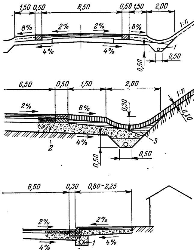
Рис. 7.17. Дренаж в дорожном строительстве [7.20]:
