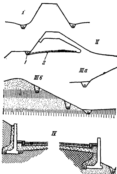
Рис. 7.15. Дренаж в подземном строительстве:
