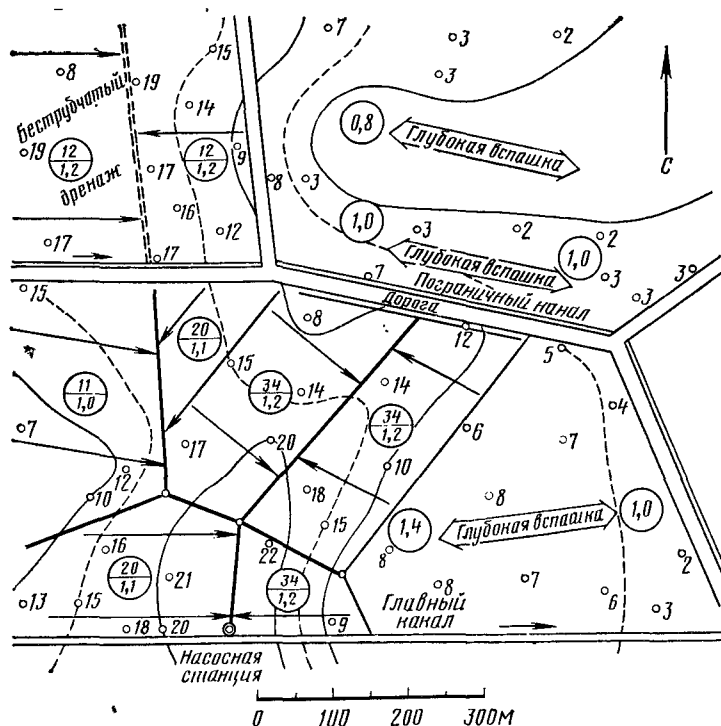
Рис. 7.24. План беструбчатого дренажа и глубокой вспашки торфяника.
