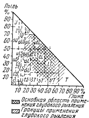
Рис. 4.7. Основная и пограничные зоны применения глубокого рыхления на минеральных почвах [4.11]:
