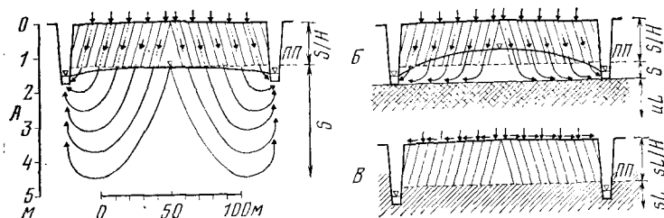
Рис. 5.18. Линии тока грунтовых вод и верховодки при глубокой вспашке [5.10]:
