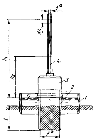
Рис. 3.16. Схема измерения инфильтрации инфильтromетром с двумя кольцами [3.22].
