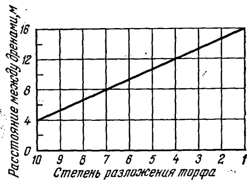
Рис. 7.20. Номограмма для определения расстояния между кротовыми дренами в торфяных почвах.
