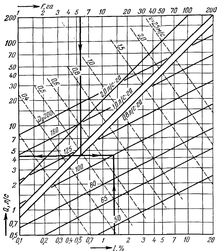
Рис. 6.2. То же, что на рисунке 6.1., но трубы гофрированные из ПВХ ( k_t=2 мм).
