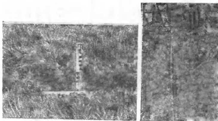
Рис. 9.14. Работа бестраншейной дренажной машины с Y-образным лемехом фирмы «Нудготак»: слева — приподнятый почвенный клин; справа — трубчатая дрена, уложенная на глубине 1,2 м. с разрыхленным почвенным клином над ней (маршевая почва).
