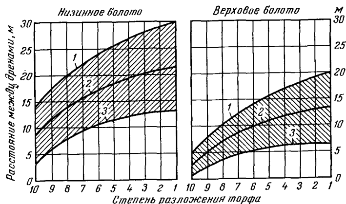
Рис. 7.12. Номограмма для определения расстояния между дренами на болотах северо-западной части ФРГ в зависимости от интенсивности предварительного осушения:
