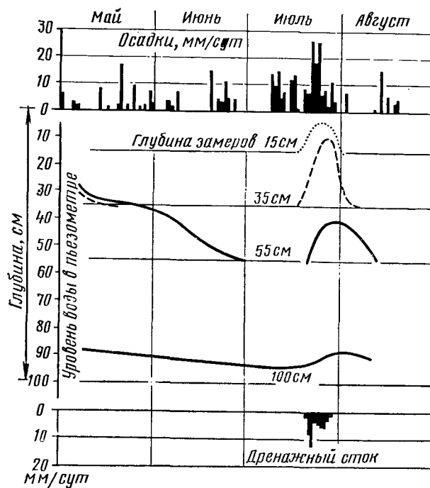
Рис. 5.16. Атмосферные осадки, верховодка и дренажный сток при комбинированном дренаже [4.7].
