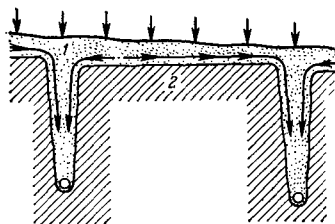
Рис. 5.5. Действие трубчатого дренажа в водопроницаемой почве [5.9]:
