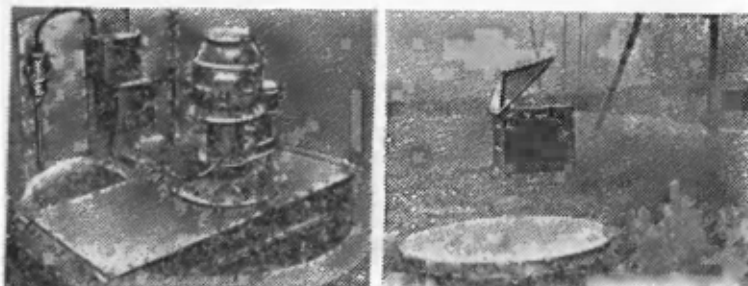
Рис. 7.2. Насосная станция перекачки дренажных вод для водосбора около 50 га.
