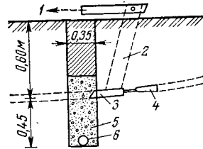
Рис. 4.3. Комбинированный дренаж [4.12]:
