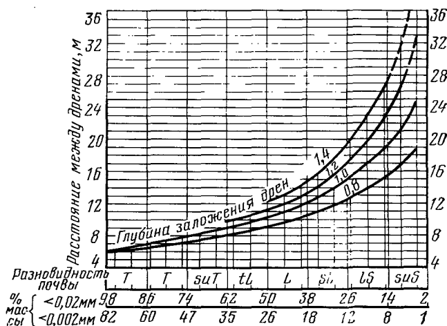
Рис. 6.10. Номограмма для определения расстояния между дренами для почв, заболоченных связанной водой. Увеличение расстояний между дренами возможно при быстром улучшении структуры почвы и уклоне поверхности более 2% [1.6]:
