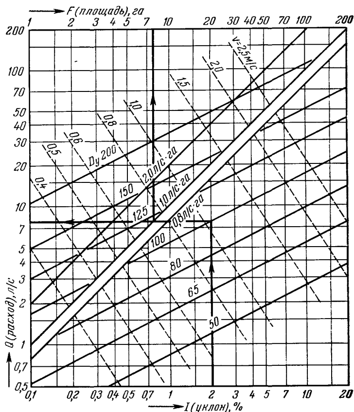
Рис. 6.1. Номограмма для определения внутреннего диаметра дрена, скорости воды и расходов. Дренажные трубы гончарные ( k_b = 0,7 мм), D_y — внутренний диаметр.
