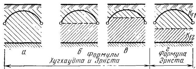
Рис. 6.8. Расположение дрен относительно поверхности соприкосновения двух слоев почвы [6.1]:
