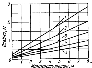
Рис. 7.10. Номограмма эмпирической формулы осадки торфа [7.25]:
