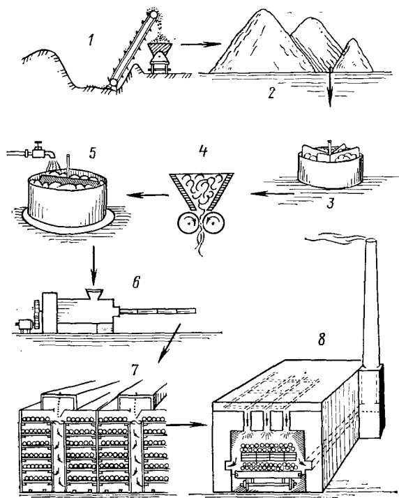
Рис. 8.1. Современное изготовление дренажных труб из глины:
