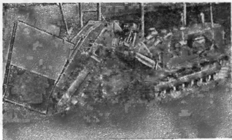
Рис. 9.5. Дренажная машина фирмы «Hoes» с фрезерно-цепным рабочим органом.
