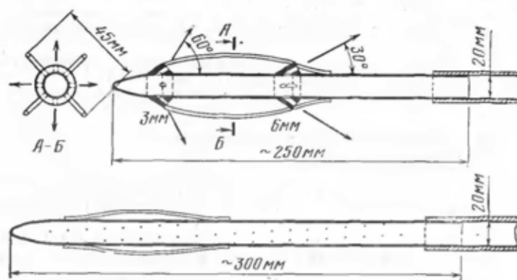
Рис. 10.2. Чертеж струйчатой трубы промывного аппарата [10.2]: сверху — для промывки назад; снизу — для промывки в сторону (масштаб не соблюден); внутренний диаметр труб 20 мм.
