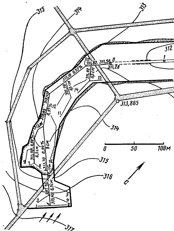
Рис. 7.23. План трубчатого дренажа долины ручья [7.31].
