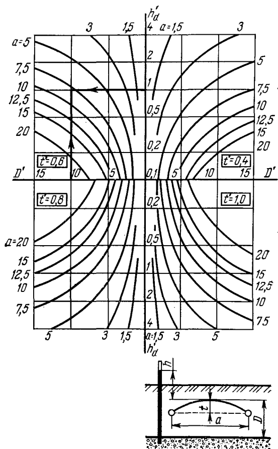
Рис. 6.12. Номограмма для определения расстояний между дренами при напорных грунтовых водах без учета атмосферных осадков [6.7].
