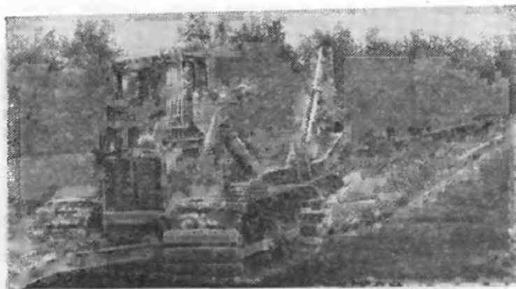
Рис. 9.20. Самоходный плуг для глубокой вспашки фирмы «Otto-teuer»; максимальная рабочая глубина 2,4 м.
