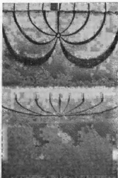
Рис. 5.1. Действие трубчатого дренажа при испытании на моделях в ящике с песком. Линии тока окрашены [5.14]:
