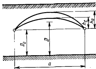
Рис. 6.14. Понижающееся зеркало грунтовых вод или переменный сток [6.1].
