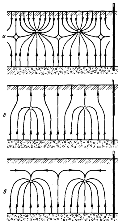
Рис. 6.11. Линии тока вод в почвах с напорными грунтовыми и поверхностными водами [6.7]:
