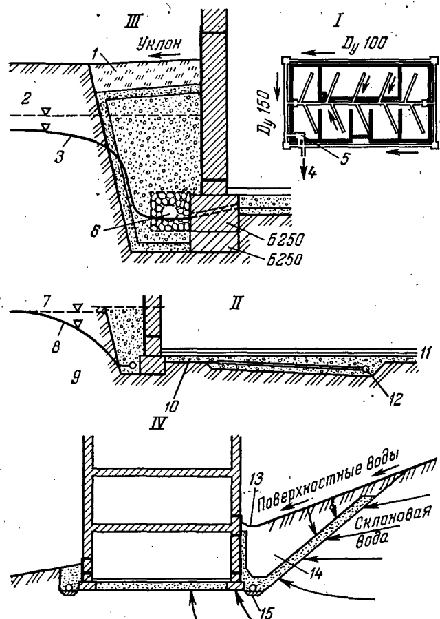
Рис. 7.18. Дренаж зданий (стандарт ФРГ DIN 4095):
