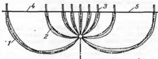
Рис. 5.2. Сравнение расчетных и окрашенных линий тока [5.14]:
