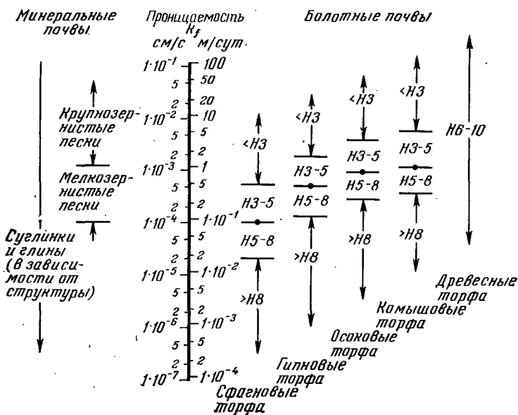
Рис. 3.14. Водопроницаемость минеральных и болотных почв [3.16].
