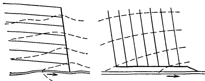
Рис. 7.5. Расположение дренажа вдоль и поперек горизонталей.
