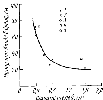
Рис. 5.14. Результаты измерения в полевых условиях сопротивления на вход в дренажные трубы при разной ширине водопропускных отверстий (щелей):
