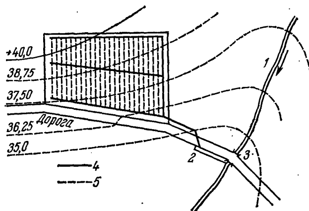
Рис. 7.21. Комбинированный дренаж:
