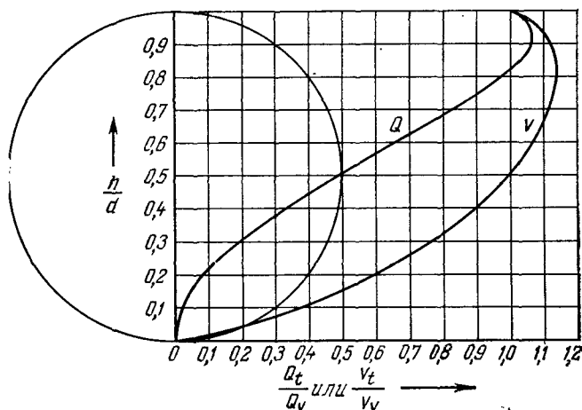
Рис. 6.4. Кривые заполнения для круглых поперечных сечений труб [6.6].
