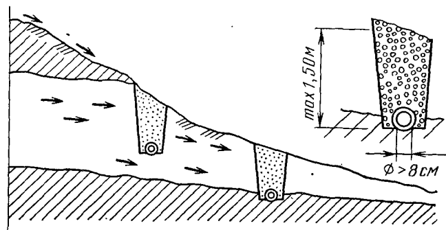
Рис. 7.7. Расположение ловчих дрен для вод, поступающих с внешних водосборных площадей (стандарт ФРГ DIN 1185, лист 1).
