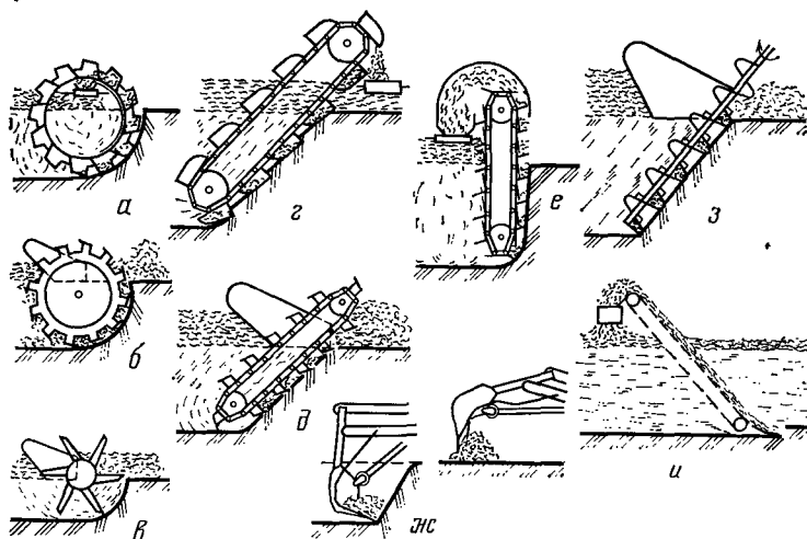
Рис. 9.2. Схемы рабочих органов различных дренажных машин:
