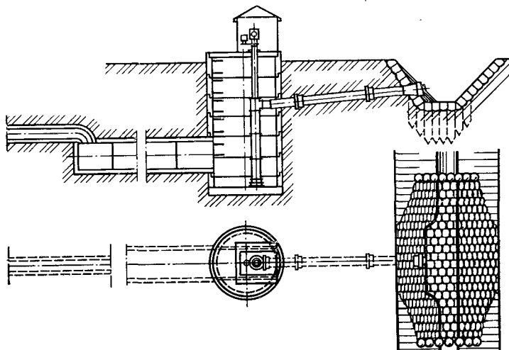
Рис. 7.1. Насосная станция перекачки дренажных вод с вертикальным насосом и электродвигателем.
