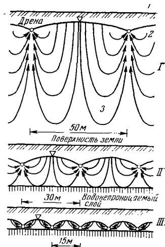
Рис. 5.4. Влияние глубины залегания водонепроницаемого слоя почвы на расстояние между дренами:
