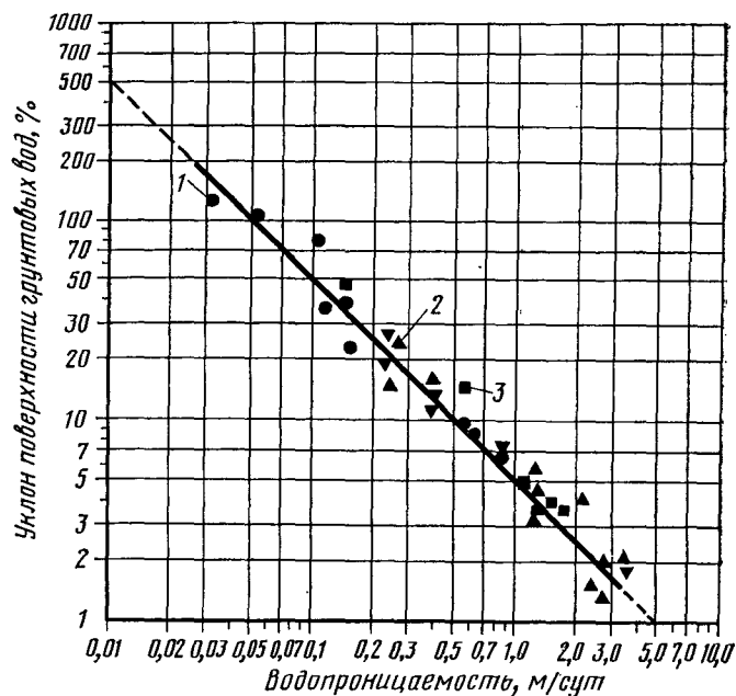
Рис. 3.11. Связь между уклоном поверхности грунтовых вод и водопрооницаемостью:
