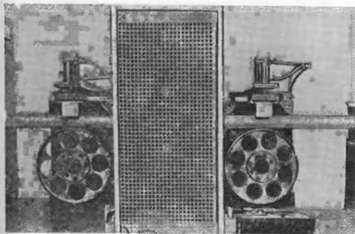
Рис. 8.7. Перфорирование дренажной трубы из ПВХ (подача справа).
