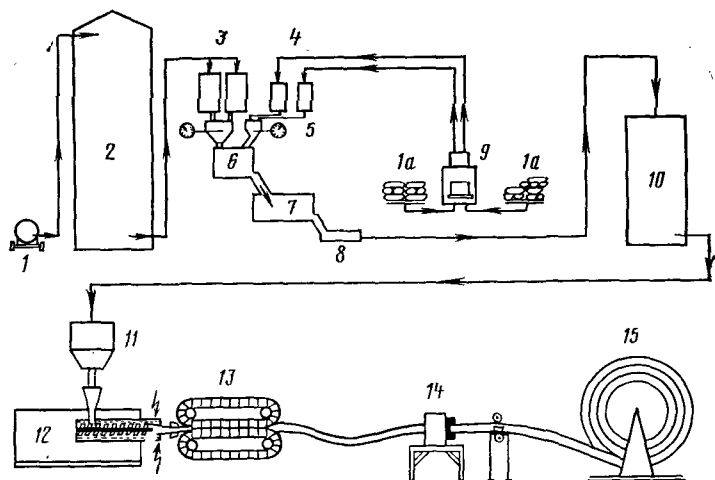
Рис. 8.5. Изготовление дренажных труб из поливинилхлорида: 1—2 — подвоз и хранение порошка ПВХ и добавок; 3—9 — дозирование, смешивание и приготовление; 10 — хранение смеси; 11—12 — воронка и экструдер; 13 — формовка труб; 14 — перфорирование; 15 — намотка труб на барабаны.
