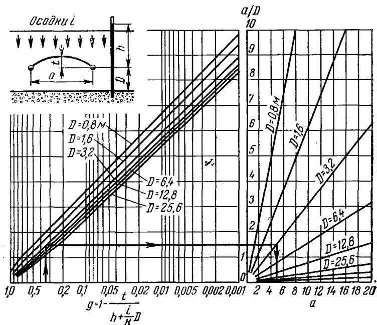
Рис. 6.13. Номограмма для определения расстояний между дренами в почвах, заболоченных напорными грунтовыми водами и водами атмосферных осадков [6.7].
