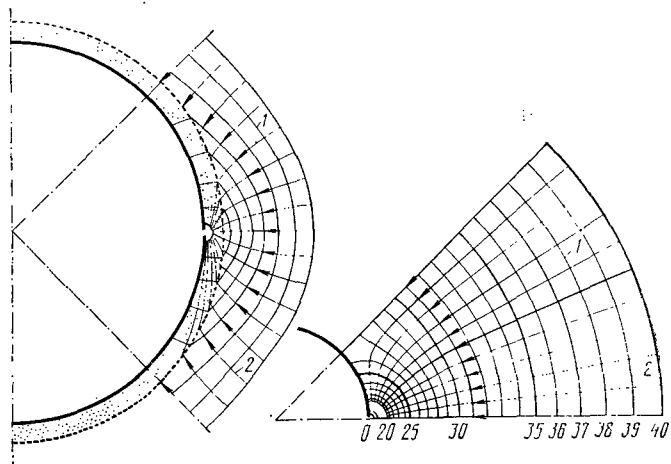
Рис. 5.11. Линия равного напора (1) и линии тока (2) воды к дренажной трубе с дренажным фильтром (левый график) и без фильтра (правый график) [5.25].
