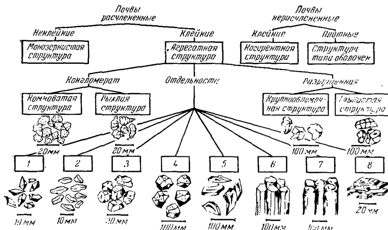
Рис. 3.6. Схема определения структуры минеральных почв [2.2]: 1 — осколочная структура; 2 — зернистая; 3 — субполиэдрическая; 4 — полиэдрическая; 5 — мелкообломочная; 6 — призматическая; 7 — столбчатая; 8 — плиточная структура.
