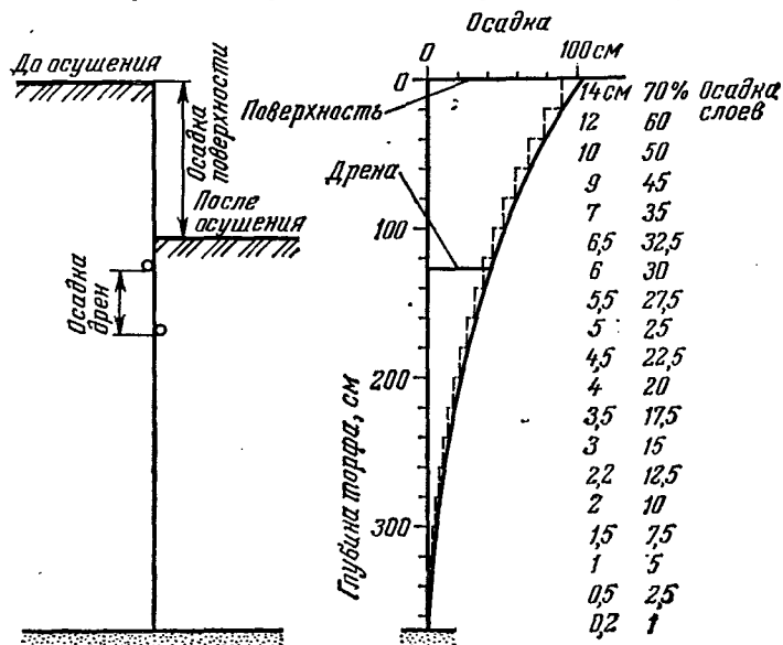
Рис. 7.11. Осадка поверхности торфа и дрен [7.3].
