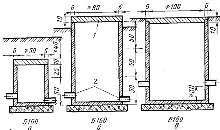
Рис. 8.26. Различные дренажные колодцы из бетонных труб [7.23]:
