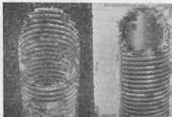
Рис. 8.11. Гофрированные дренажные трубы из ПВХ: слева — без наклеенной изнутри пленки, справа — с наклеенной изнутри пленкой.
