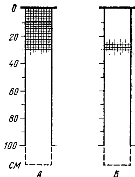
Рис. 4.5. Механическое уплотнение верхнего слоя почвы (стандарт ФРГ DIN 1185, лист. 1):
