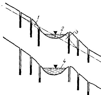
Рис. 3.9. Разрез на местности с грунтовыми и поверхностными водами [3.9]:
