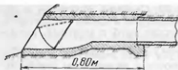
Рис. 8.22. Дренажное устье для коллектора из бетона с решетчатым клапаном [7.23].
