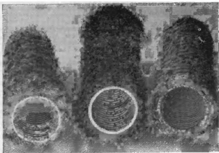
Рис. 8.16. Пластмассовые дренажные трубы, обернутые в фильтрующие материалы: слева направо — кокосовое волокно, полипропиленовое волокно и флътан из дуо (верхний слой) + торфяное волокно (внутренний слой).
