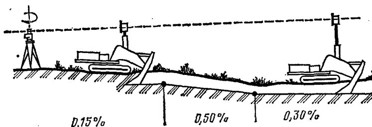
Рис. 9.4. Автоматическое управление высотой (включая изменение уклона) с помощью лазерной системы.
