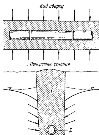
Рис. 5.7. Действие дрены при низкой водопроницаемости засыпки дренажной траншеи [5.9]:
