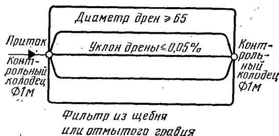
Рис. 7.19. Трубчатый дренаж для поверхностных самотечных поливов осветленными сточными водами, поступающими из жилых домов на одну—две семьи.
