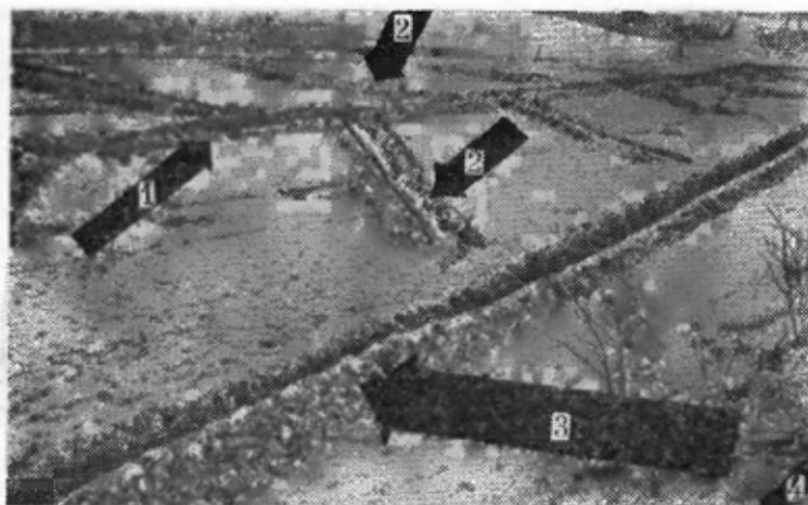
Рис. 4.1. Коллектор (1), всасывающая (регулирующая) дрена (2) и ловчая дрена (3). Последняя принимает грунтовый поток со склона (4) и отводит его [4.5].
