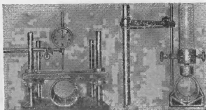
Рис. 8.9. Испытания дренажной трубы из ПВХ на сжатие и ударную прочность.
