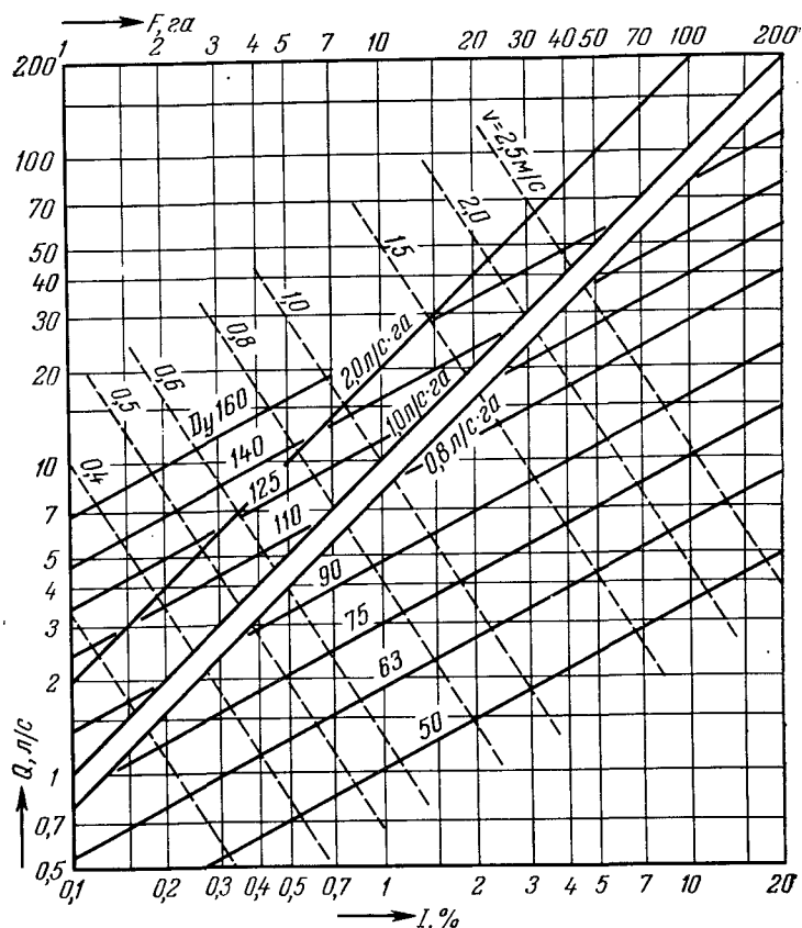
Рис. 6.3. То же, что на рисунке 6.1., но трубы гладкие из ПВХ ( k_b=0,1 мм).
