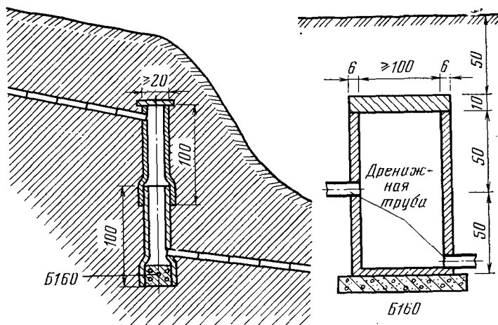
Рис. 8.27. Дренажный перепад [7.23].
