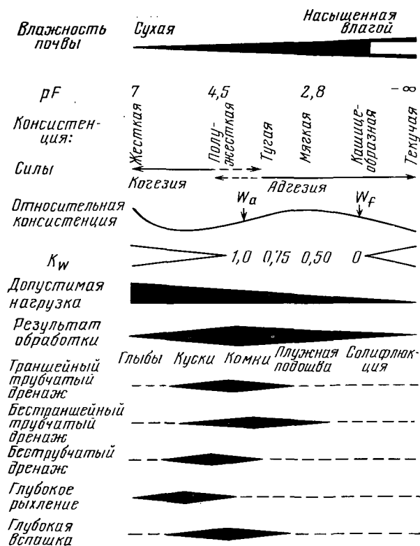
Рис. 9.1. Свойства связанных почв в зависимости от их влажности и возможности применения дренажных машин (по неопубликованным материалам проф. Х. Куптце).
