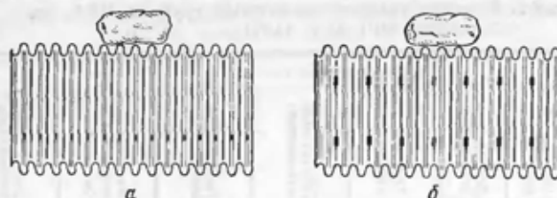
Рис. 8.10. Расположение водовпускных отверстий в гофрированных дренажных трубах из ПВХ.
