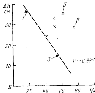
Рис. 5.19. Корреляция сопротивления на вход воды в дрена при свободных водовыпускных отверстиях дренажных труб из ПВХ [5.11]:
