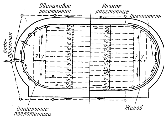
Рис. 7.13. Дренаж спортивных площадок (стандарт ФРГ DIN 18035).
