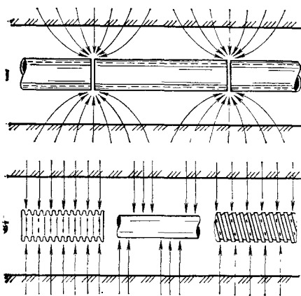
Рис. 5.8. Поступление воды в дренажную гончарную трубу (А) и трубу из ПВХ (Б).
