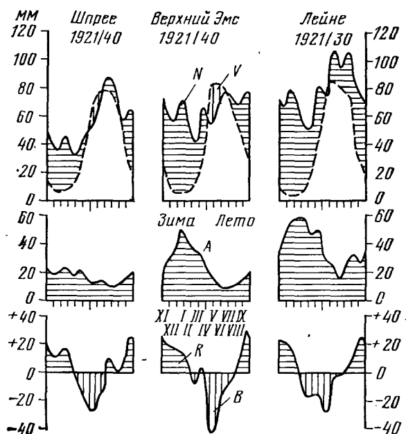
Рис. 2.2. Среднегодовые колебания водного баланса рек Шпрее, Верхний Эмс и Лейне (Вюртемберг) [2.1].
