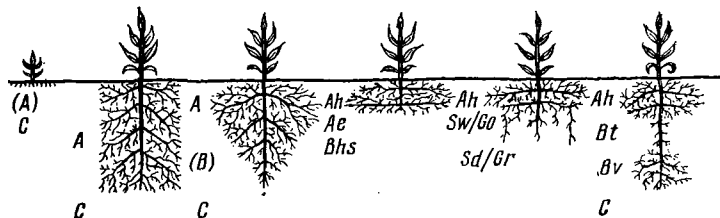
Рис. 3.19. Распространение корней в зависимости от типа и структуры почвы [2.2]:
