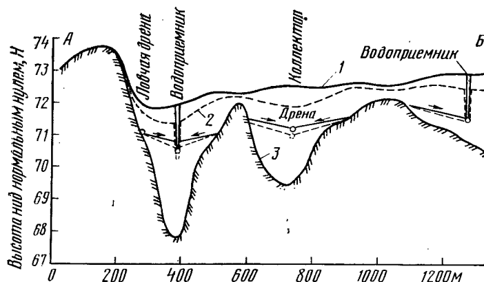
Рис. 3.3. Разрез местности по А—Б (см. рис. 3.2) до и после дренаживания [3.2]:
