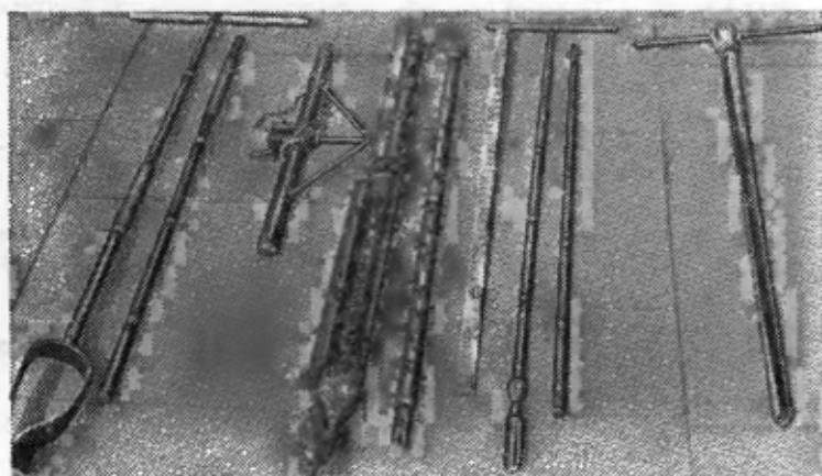
Рис. 3.1. Ручной буровой инструмент со штангами. Слева направо: лопастной бур, камерный бур, ложечный бур для промера минерального дна болота, желобчатый бур.
