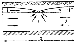
Рис. 6.5. Вертикальные, горизонтальные и радиальные компоненты течения в водопроницаемой почве над водонепроницаемым слоем [6.1]: 1 — радиальное течение; 2 — вертикальное течение; 3 — горизонтальное течение.
