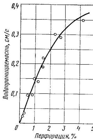
Рис. 5.9. Водопроницаемость гофрированных дренажных труб из ПВХ в зависимости от их перфорации [5.16].
