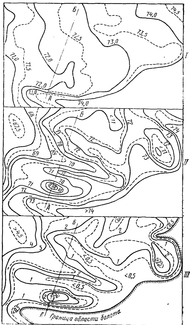
Рис. 3.2. План поверхности болота [3.2]. Разрез А—Б на рисунках 3.3 и 3.7:
