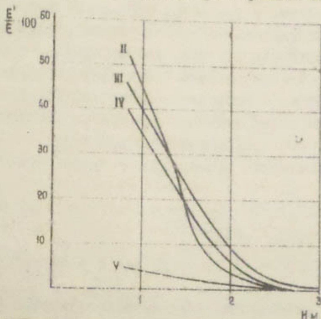
Рис.3. Зависимость доли участия грунтовых вод в формировании суммарного испарения от глубины их залегания. (II, III, IV, V — гидромодульные районы). (по В.Р. Шредеру)
