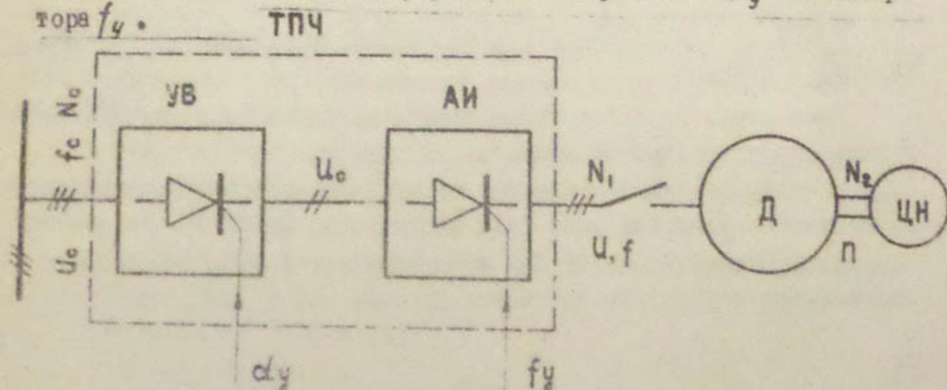
Рис. 2. Схема регулирования производительности насоса посредством ТПЧ.
