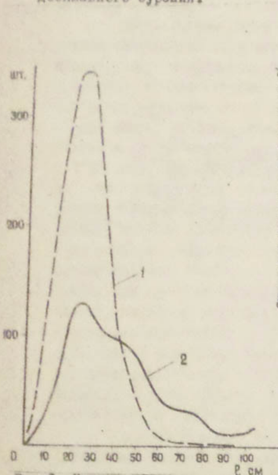
Рис.3. Кривые абсолютного распределения плашек керна по их длине при бурении твердосплавными (1) и алмазными (2) коронками.
