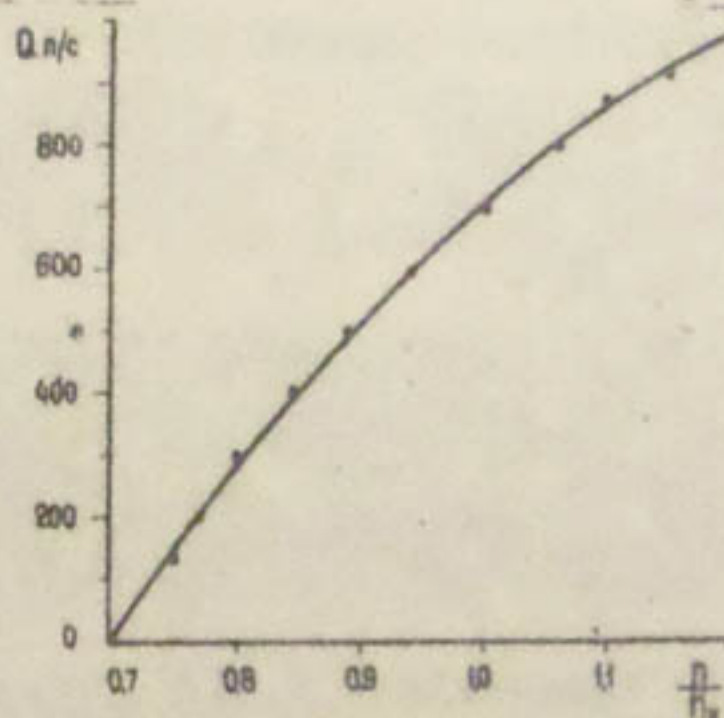
Рис. 3. Регулировочная характеристика насоса.
