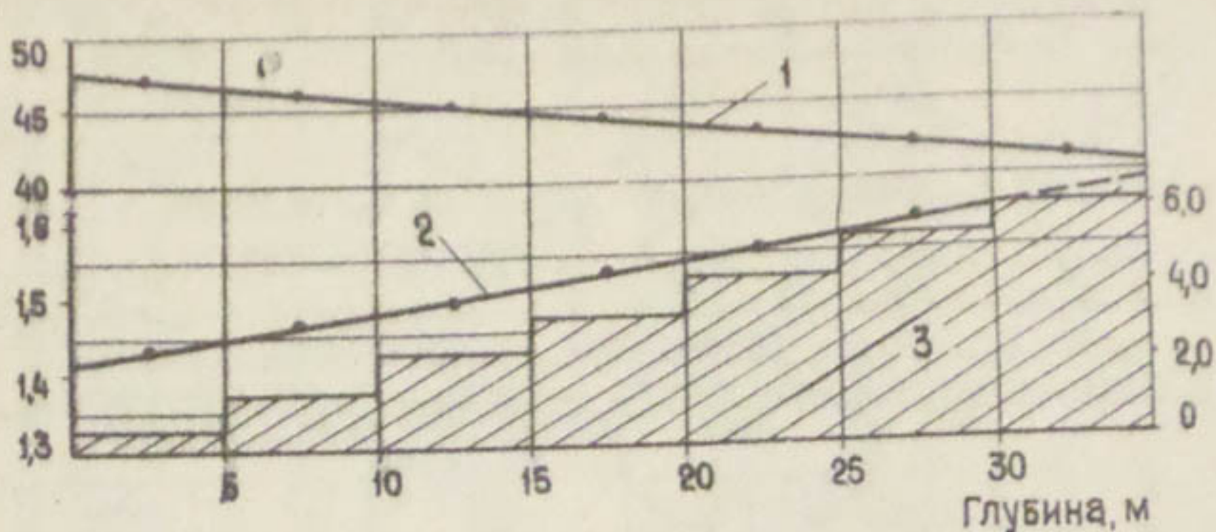
Рис. 2. Изменение плотности лесса по зонам после длительного замачивания: 1 - пористость, %; 2 - объемная масса скелета грунта, т/м³; 3 - эпюры средних напряжений в просадочной породе при ее замачивании, кгс/см².
