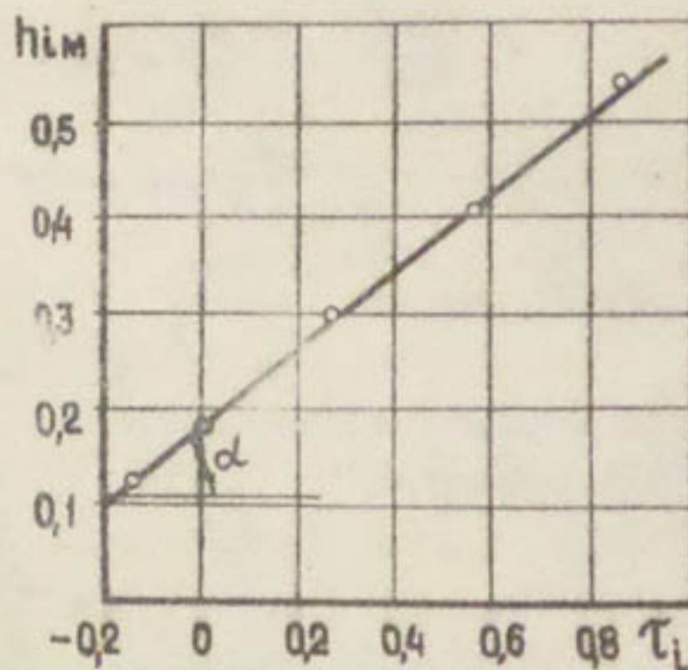
Рис. 4. Зависимость h_i = f(\tau_i) , полученная в опытах с фильтром из технического капрона.
