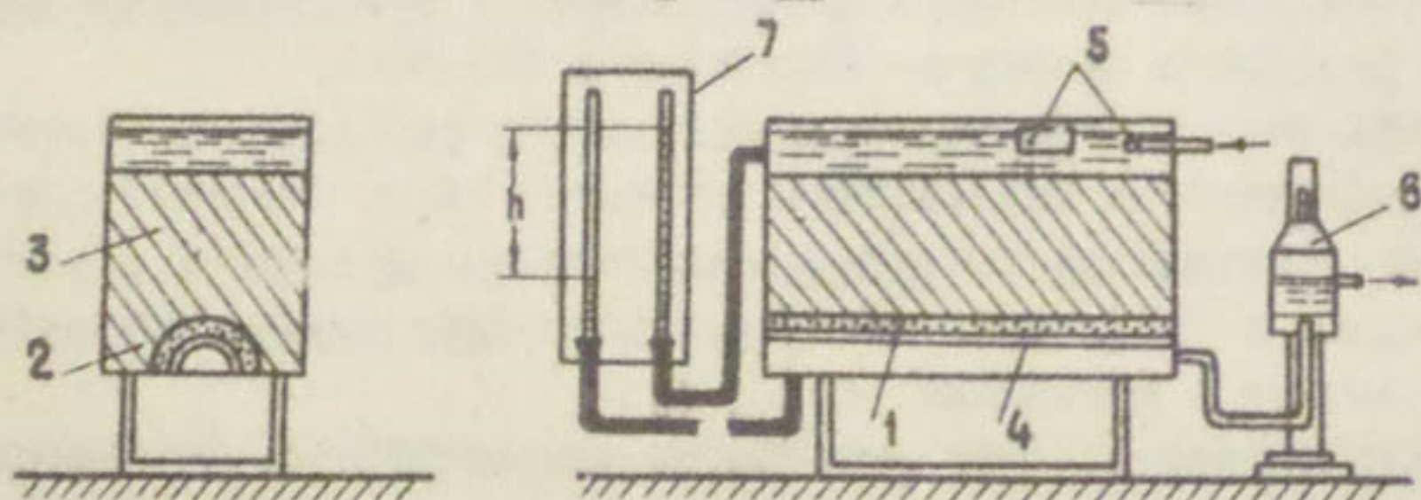
Рис. 1. Схема проведения опыта в прямоугольном фильтрационном лотке:
