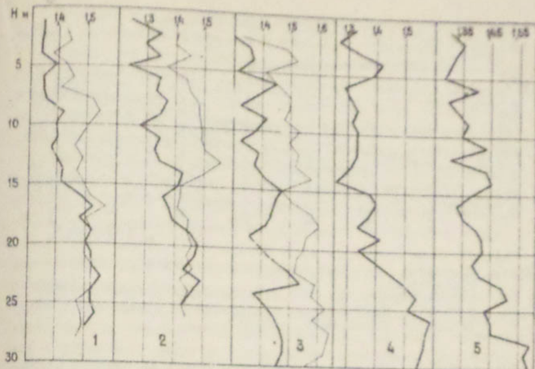
Рис. 1. Изменение объемной массы скелета лесса с глубиной (--- до замачивания, — после замачивания): 1 - опытный котлован № 1 в Каршинской степи; 2 - опытный котлован № 1 на Кок-Аральском массиве; 3 - Северный Ташкентский канал; 4 - перепадная ГЭС; 5 - Самаркандская котловина, шурф 92.
