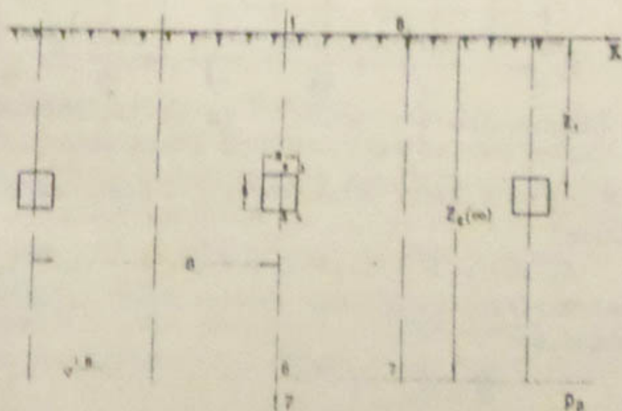
Рис. 1. Расчетная схема к задаче влагопереноса при ВПО.
