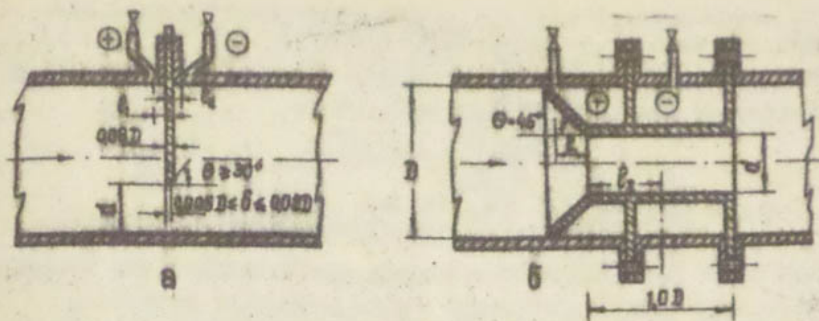
Рис. 1. Схемы исследованных конструкций водомерных устройств:
