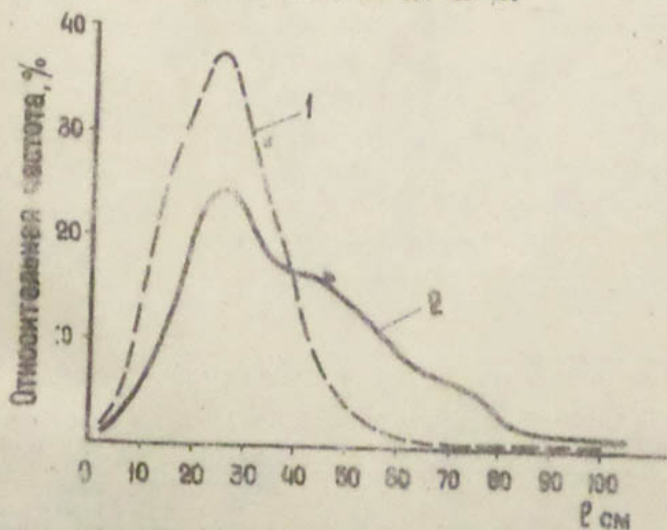
Рис. 2. Кривые относительных частот длины плашек керн при бурении твердосплавными (1) и алмазными (2) коронками при глубине скважин более 15 м.
