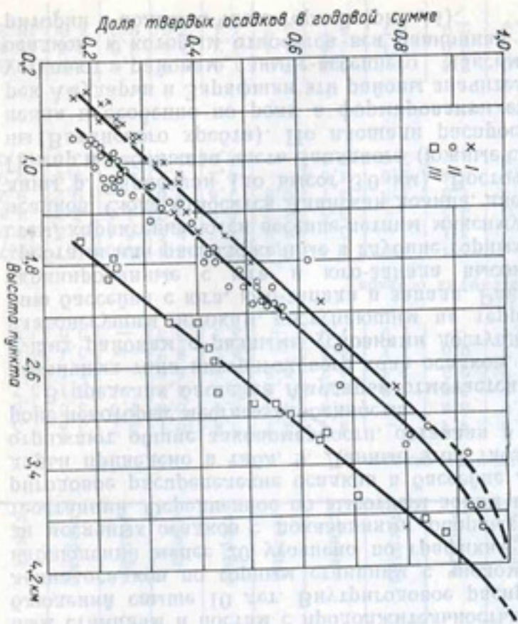
Рис. 18. Зависимость относительной доли твердых осадков в головной сумке от высоты места.
