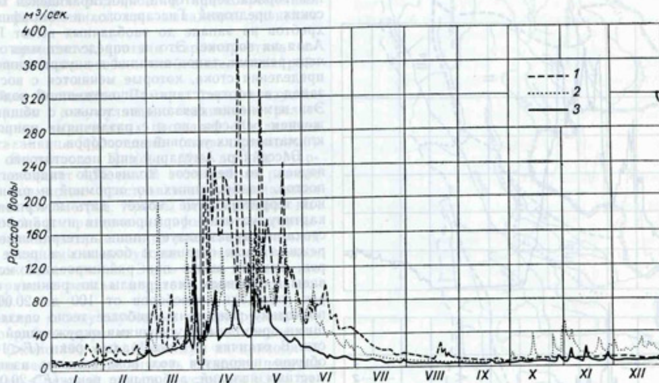
Рис. 33. Гидрограф стока р. Яхсу у кишл. Карбостонак за характерные по водности годы. 1 — многоводный (1949), 2 — средний (1953), 3 — маловодный (1947).
