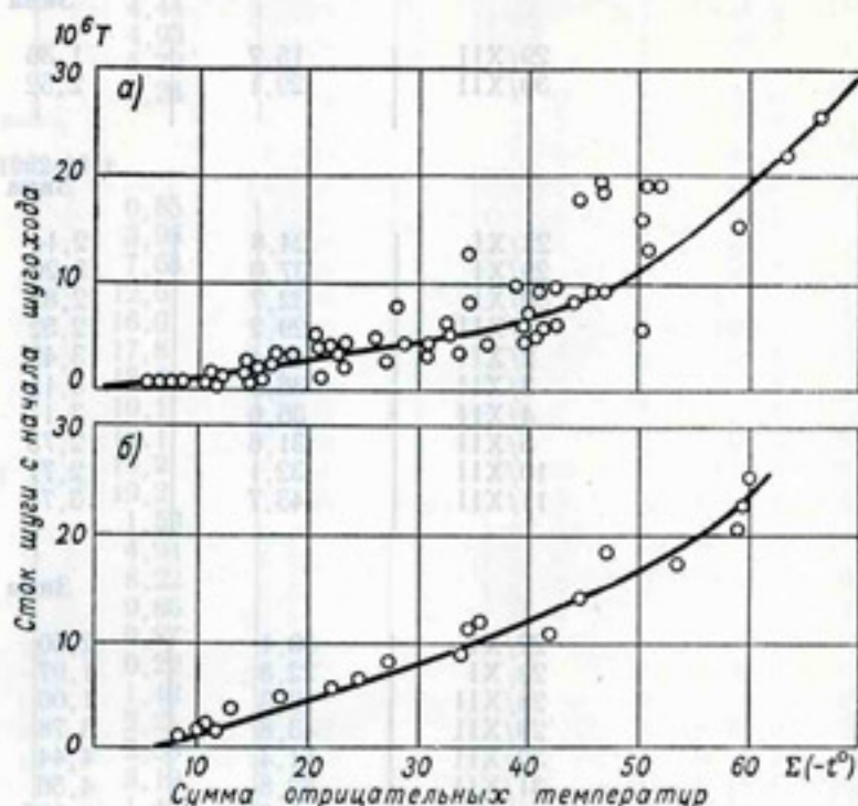
Рис. 131. Зависимость величины стока шуги за шугоход от суммы отрицательных температур для постов Чатлы (а) и Тюмюн (б).
