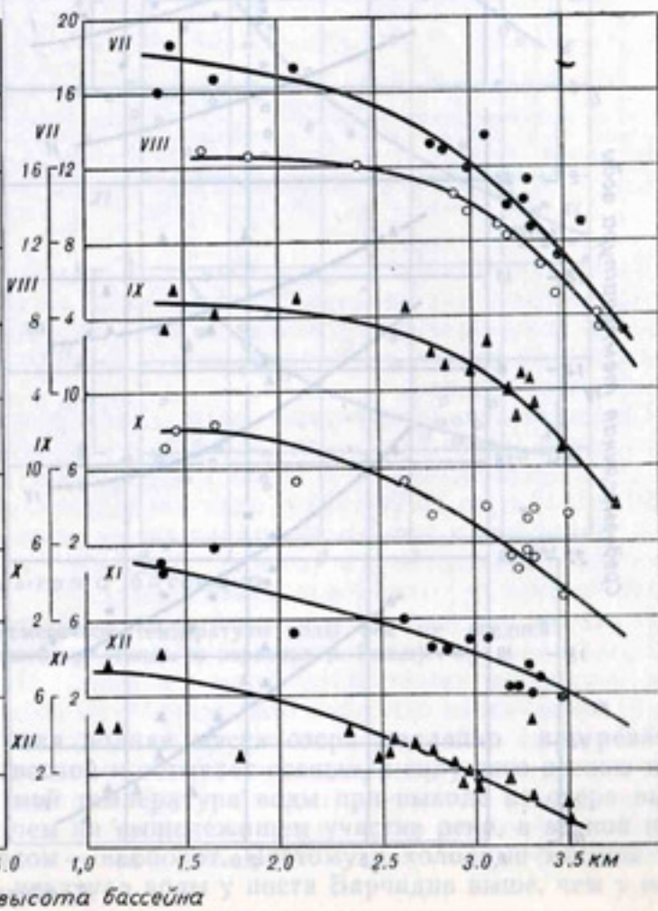
Рис. 86. Зависимость средней многолетней среднемесячной температуры воды рек от средней высоты бассейнов для рек района V (бассейн р. Зарафшан).
