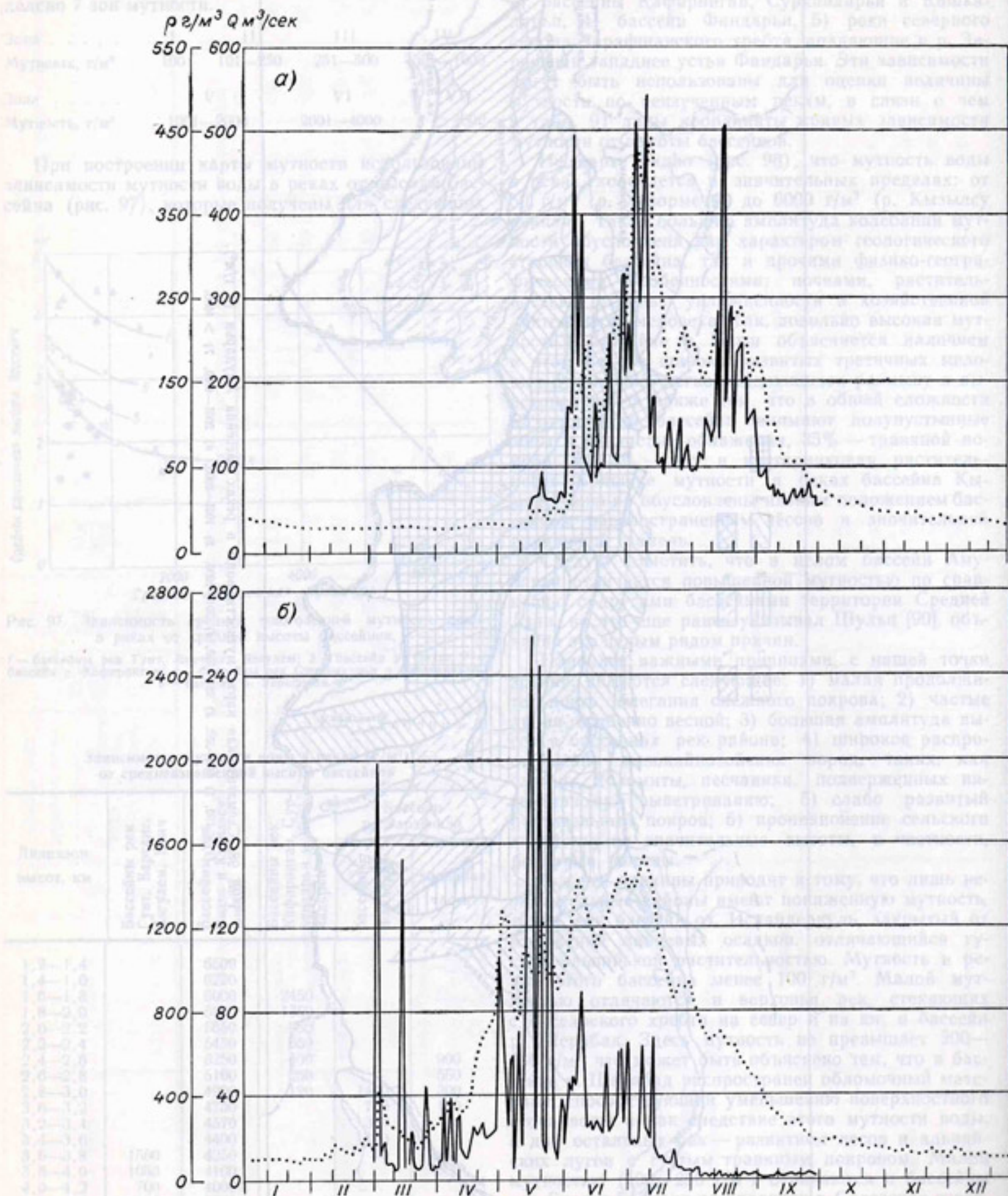
Рис. 99. Хронологические графики хода а — р. Гунт — г. Хорог, б — р. Варзоб — кишл. Даганата.
