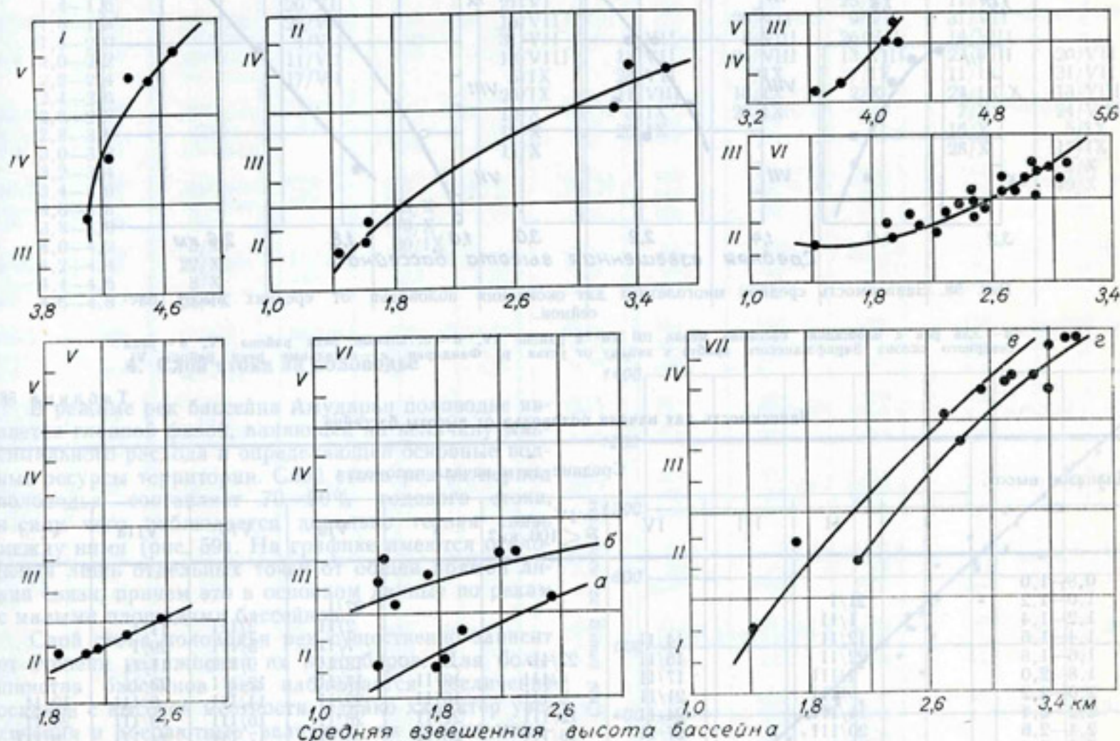
Рис. 57. Зависимость средних многолетних дат начала половодья от средних высот бассейнов для рек бассейна Амударья.
