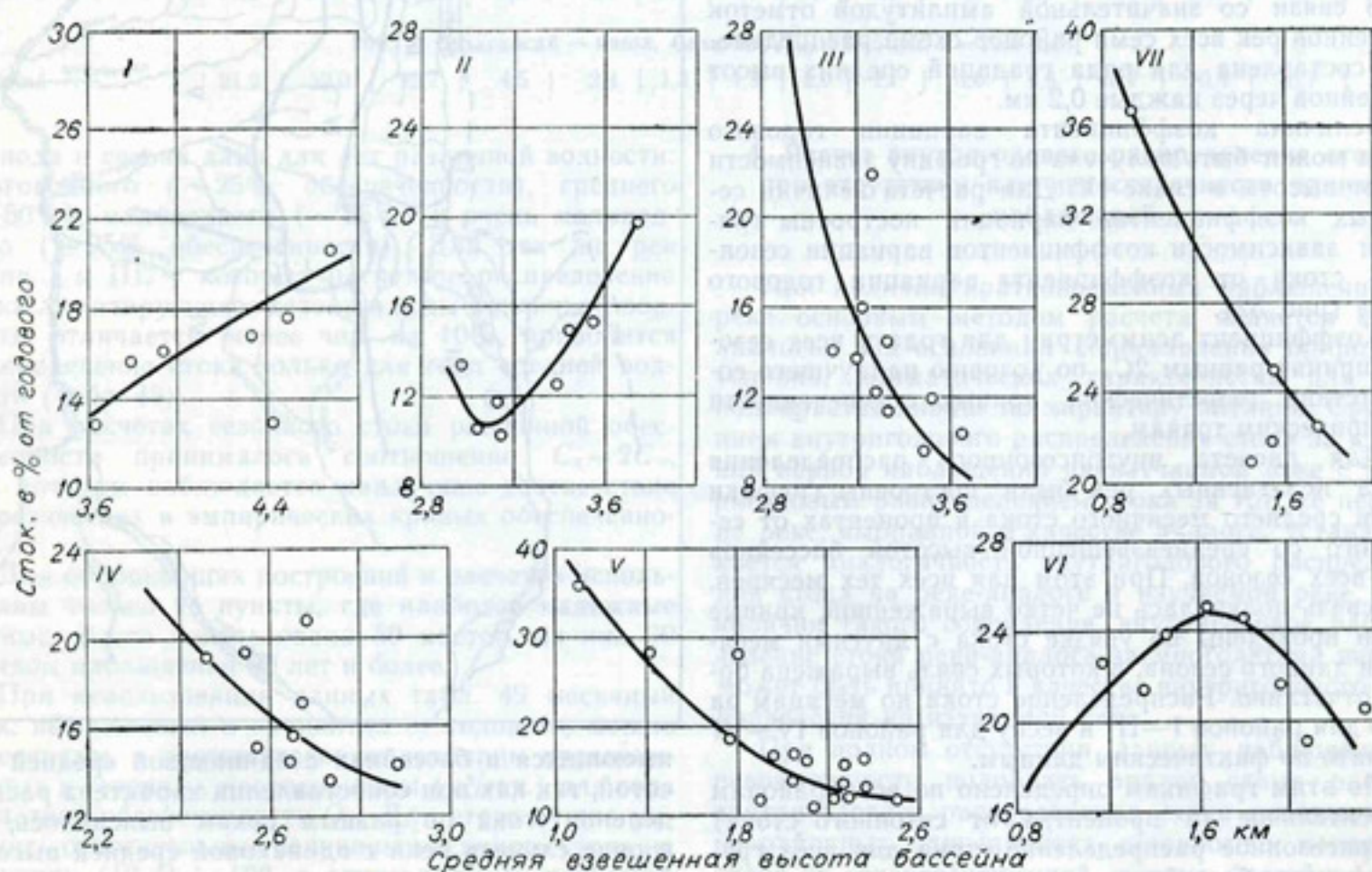
Рис. 50б. Зависимость стока за нелимитирующий сезон (в % от годового) от средней взвешенной высоты бассейнов.
