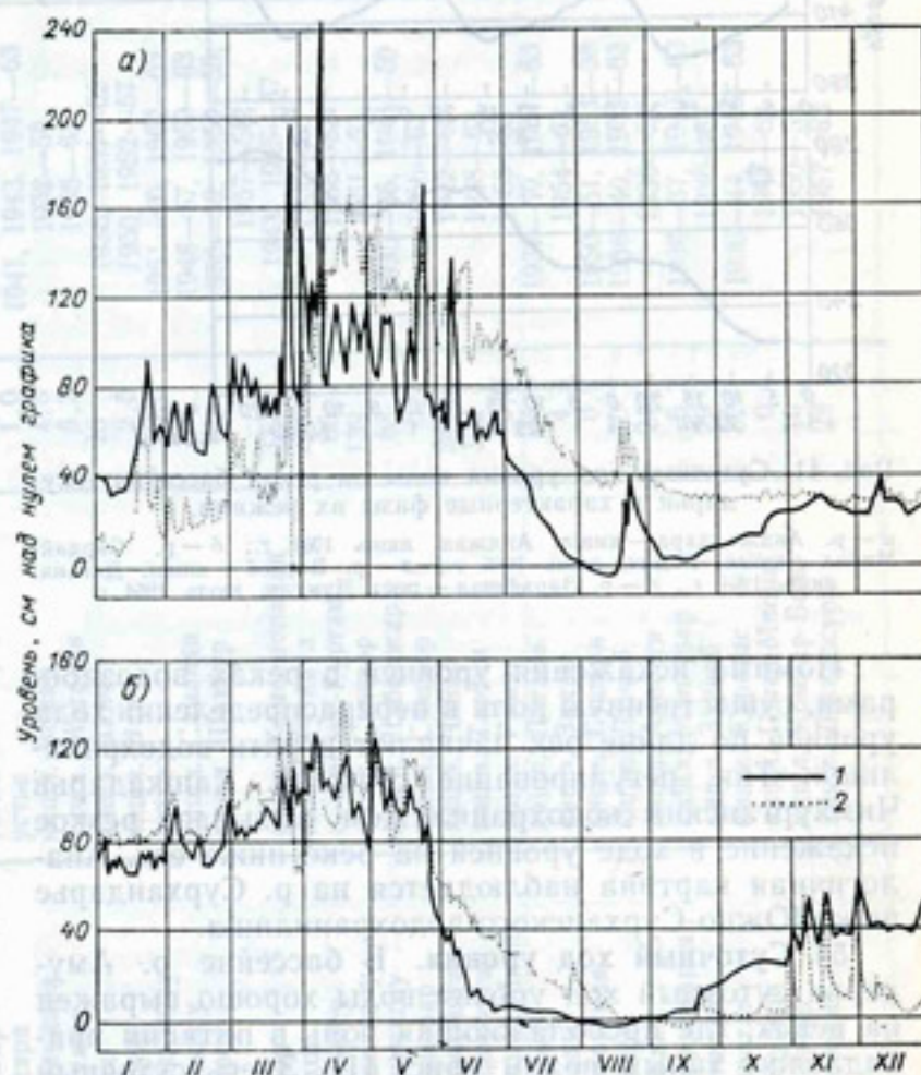
Рис. 40. Годовой ход уровня воды в р. Яхсу на постах выше (1 — кишл. Карбозтонак) и ниже (2 — пгт им. Восте) за многоводный 1949 (а) и маловодный 1947 (б) годы.
