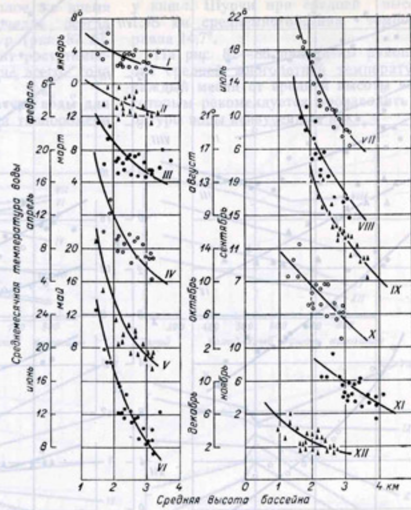
Рис. 83. Зависимость средней многолетней среднемесячной температуры воды рек от средней высоты бассейнов для рек района II (бассейн р. Кафирниган и нижняя часть бассейна р. Вахш).
