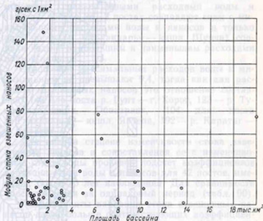
Рис. 94. Зависимость среднего многолетнего модуля стока взвешенных наносов от площади бассейна.
