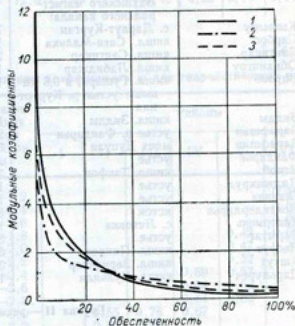
Рис. 53. Средние кривые продолжительности средних суточных расходов рек различных групп.
