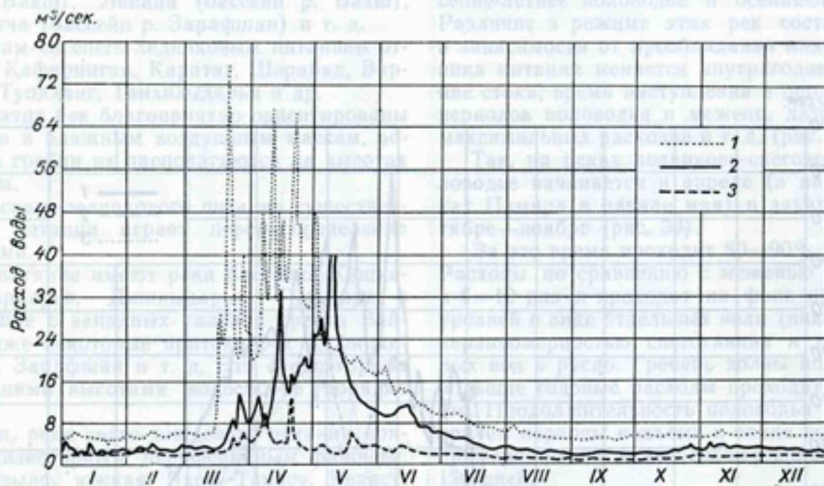
Рис. 32. Гидрограф стока р. Гузардары у кишл. Яртепа за характерные по водности годы.
