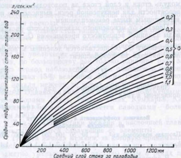
Рис. 68. Номограмма для определения среднего модуля максимального стока талых вод.
