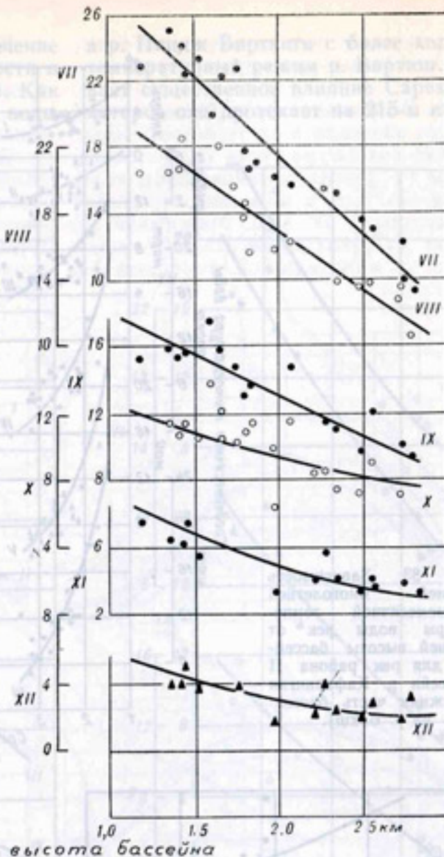
Рис. 85. Зависимость средней многолетней среднемесячной температуры воды рек от средней высоты бассейнов для района IV (бассейны рек Шерабад и Кашкадарьи).
