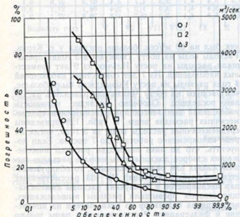
Рис. 123. График обеспеченности относительных ошибок вычисления среднемесячных расходов на постах р. Амударьи (1) и кривые обеспеченности среднемесячных расходов по постам Керки (2) и Чатлы (3).
