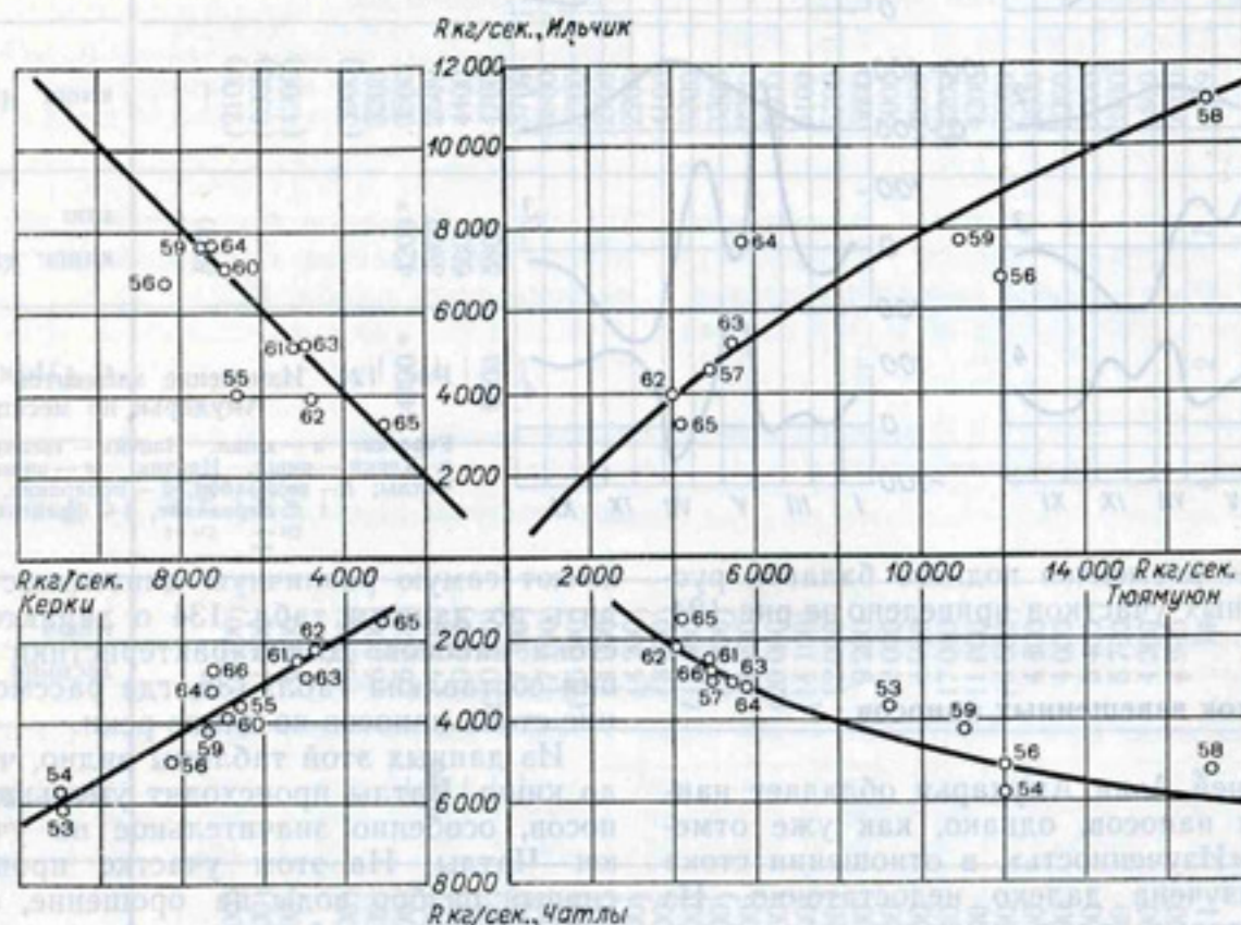
Рис. 125. Графики связи среднегодовых расходов взвешенных наносов по постам р. Амударьи.
