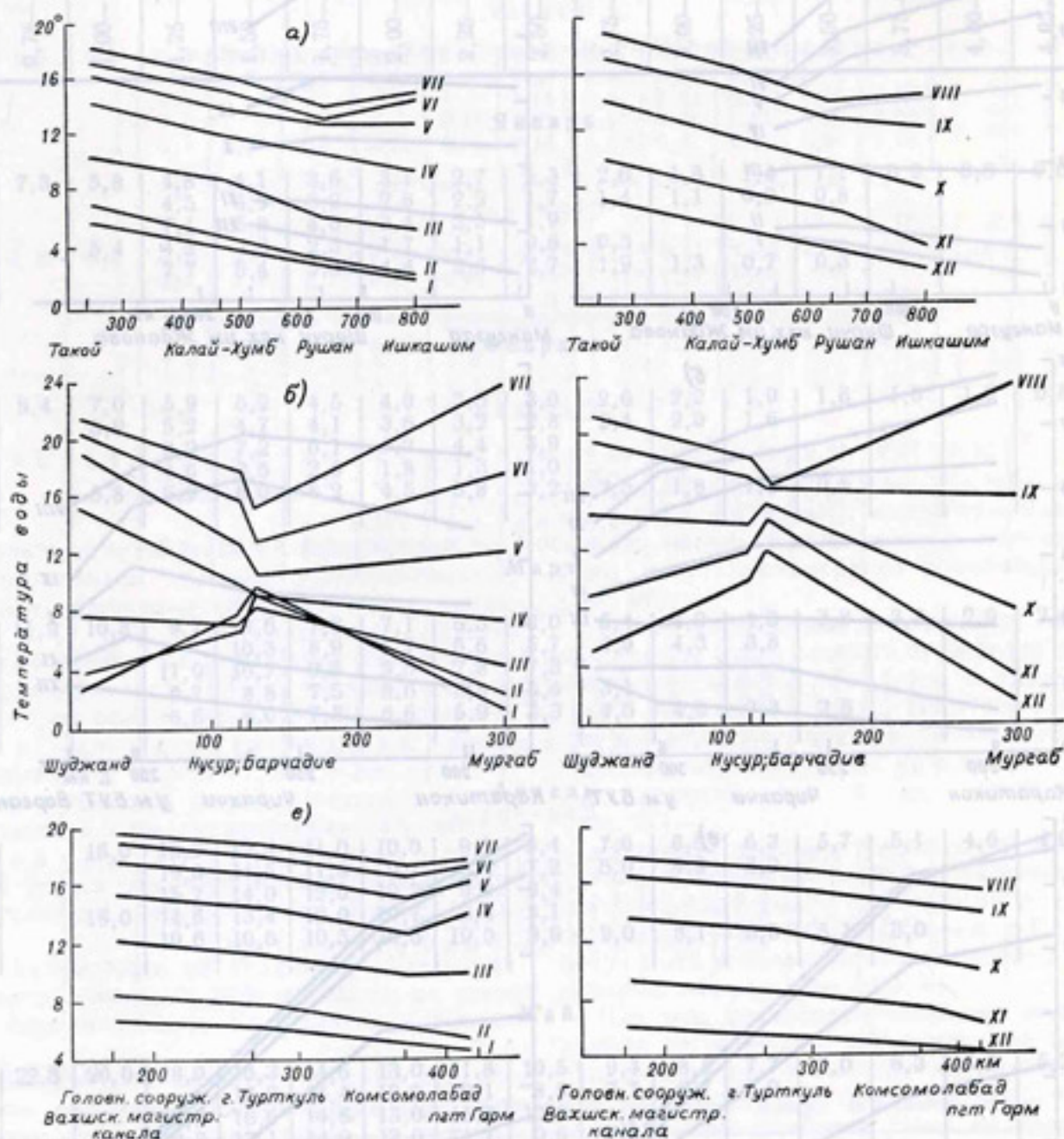
Рис. 87. Изменение среднемесечной температуры воды по длине рек Пяндж (а), Бартаг (б) и Вахш (в) (расстояние — от устья).
