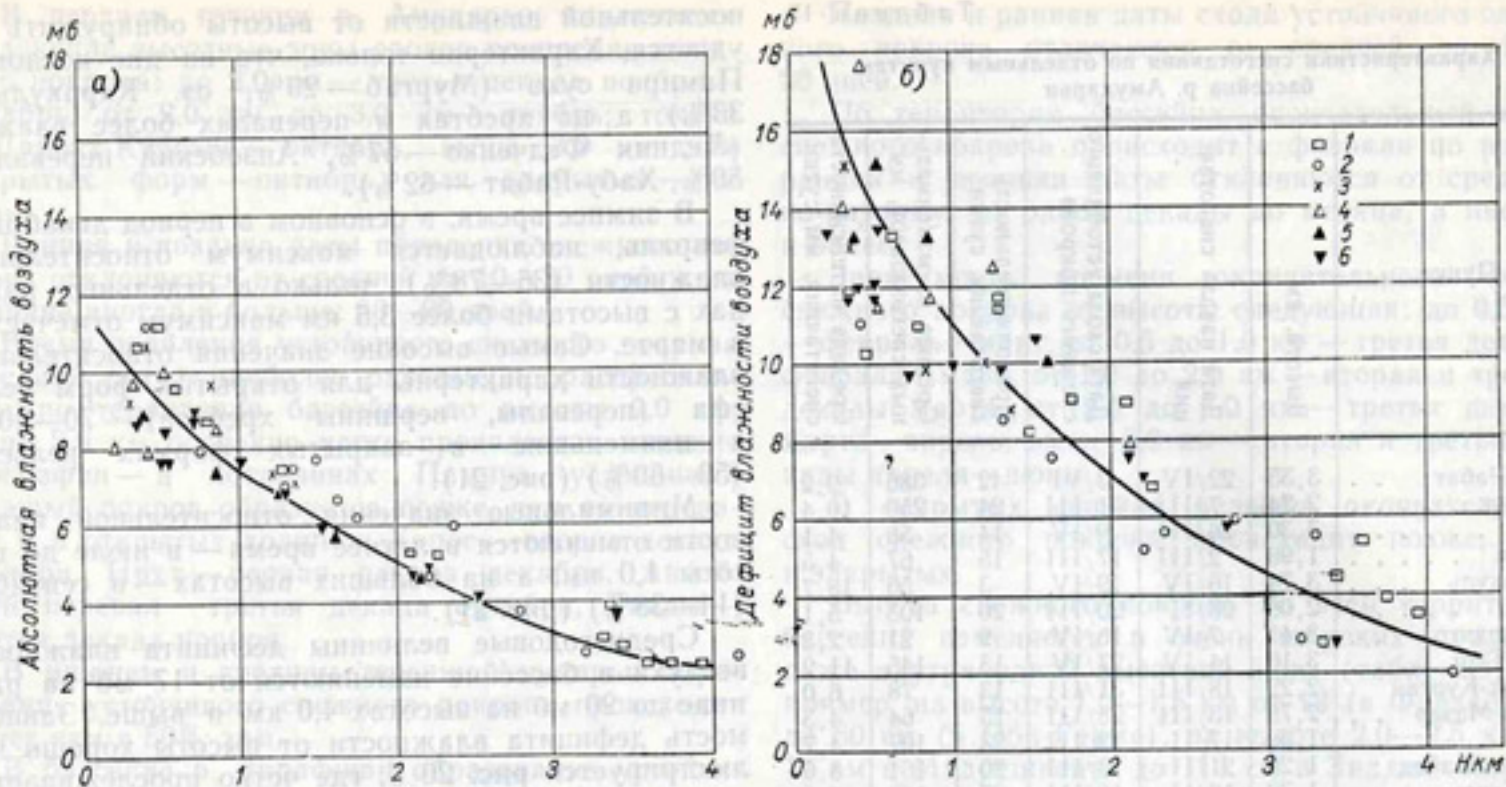
Рис. 20. Зависимость абсолютной влажности (а) и дефицита влажности (б) воздуха от высоты места. 1 — бассейны р. Пяндж, 2 — бассейны р. Вахш, 3 — бассейны р. Кафирниган, 4 — бассейны р. Сурхандарьи, 5 — бассейны р. Кашкадарьи, 6 — бассейны р. Зарафшан.
