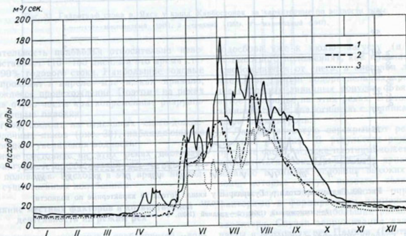
Рис. 30. Гидрограф стока р. Язгулем у кишлака Мотрави за характерные по водности годы.
