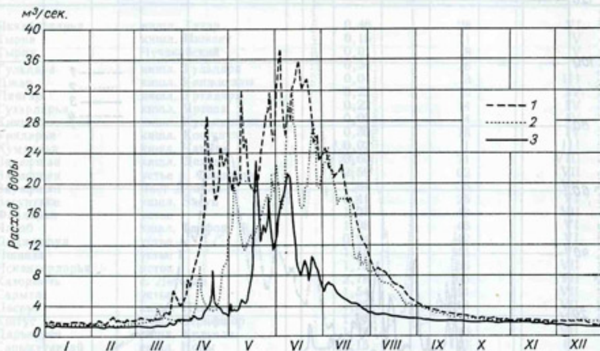
Рис. 31. Гидрограф стока р. Яккабагары у кишл. Татар за характерные по водности годы.
