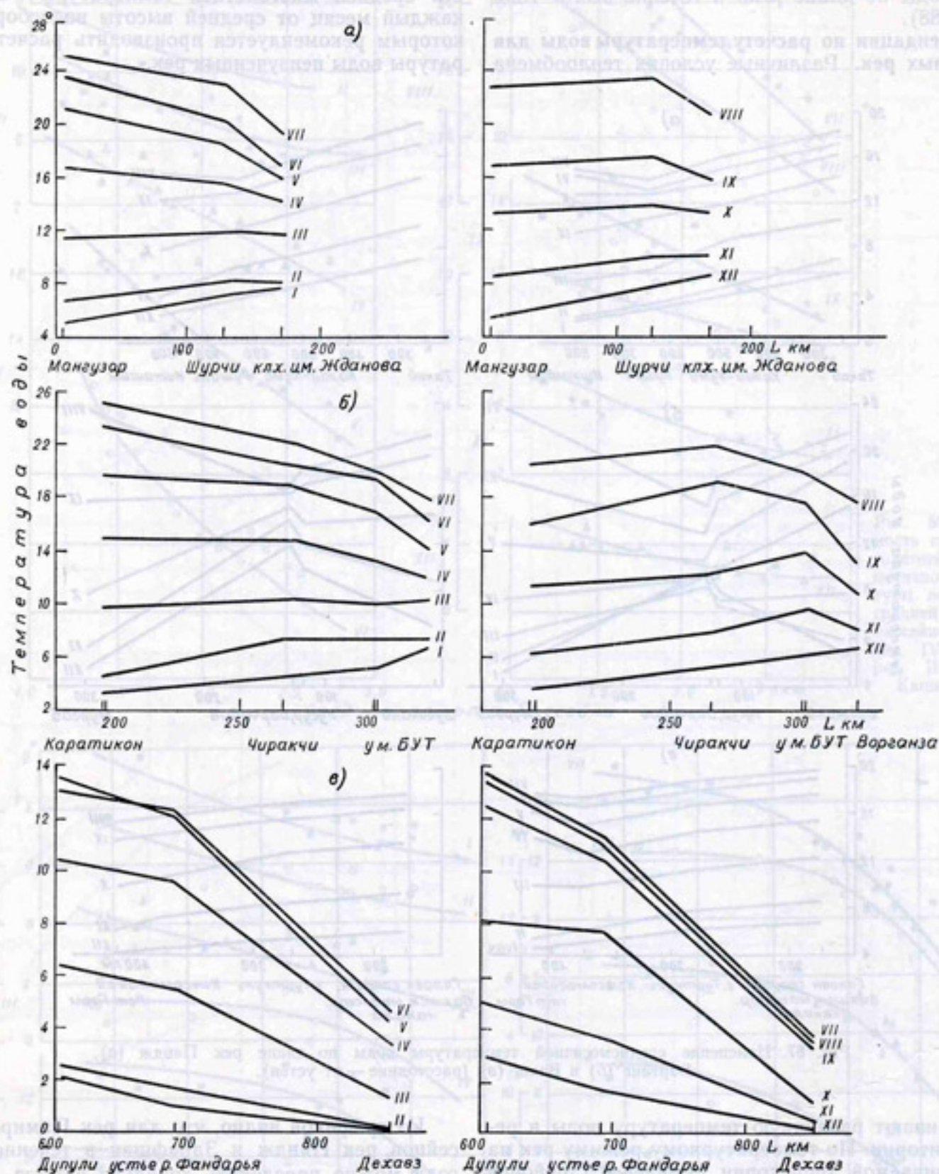
Рис. 88. Изменение среднемесячной температуры воды по длине рек Сурхандарьи (а), Кашкадарьи (б) и Зарафшан (в).
