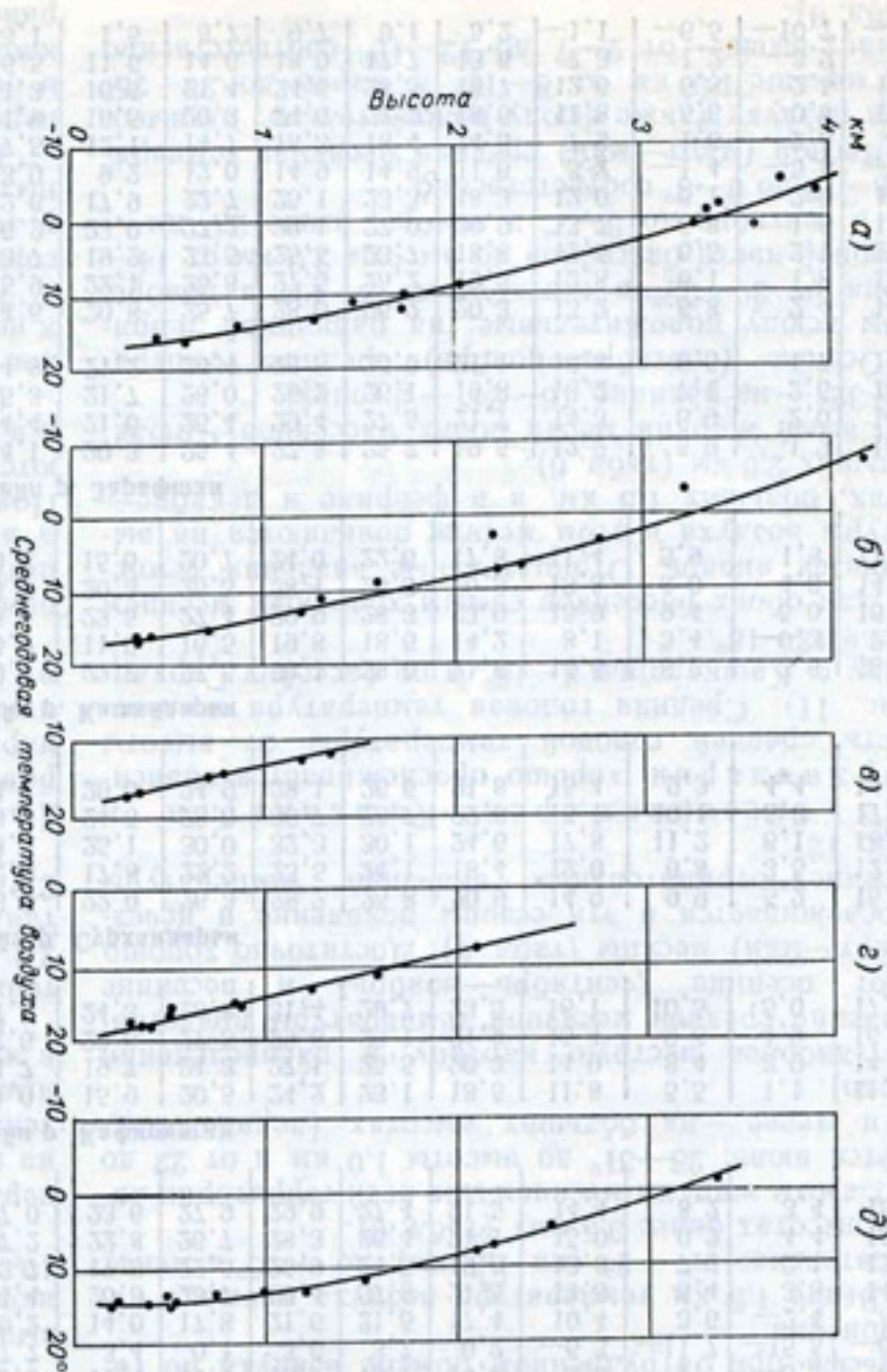
Рис. 11. Зависимость среднегодовой температуры воздуха от высоты места в бассейнах рек Пинджа (а), Вахша (б), Кафирнигана (в), Сурхандарьи (д), Зарафшана (е).
