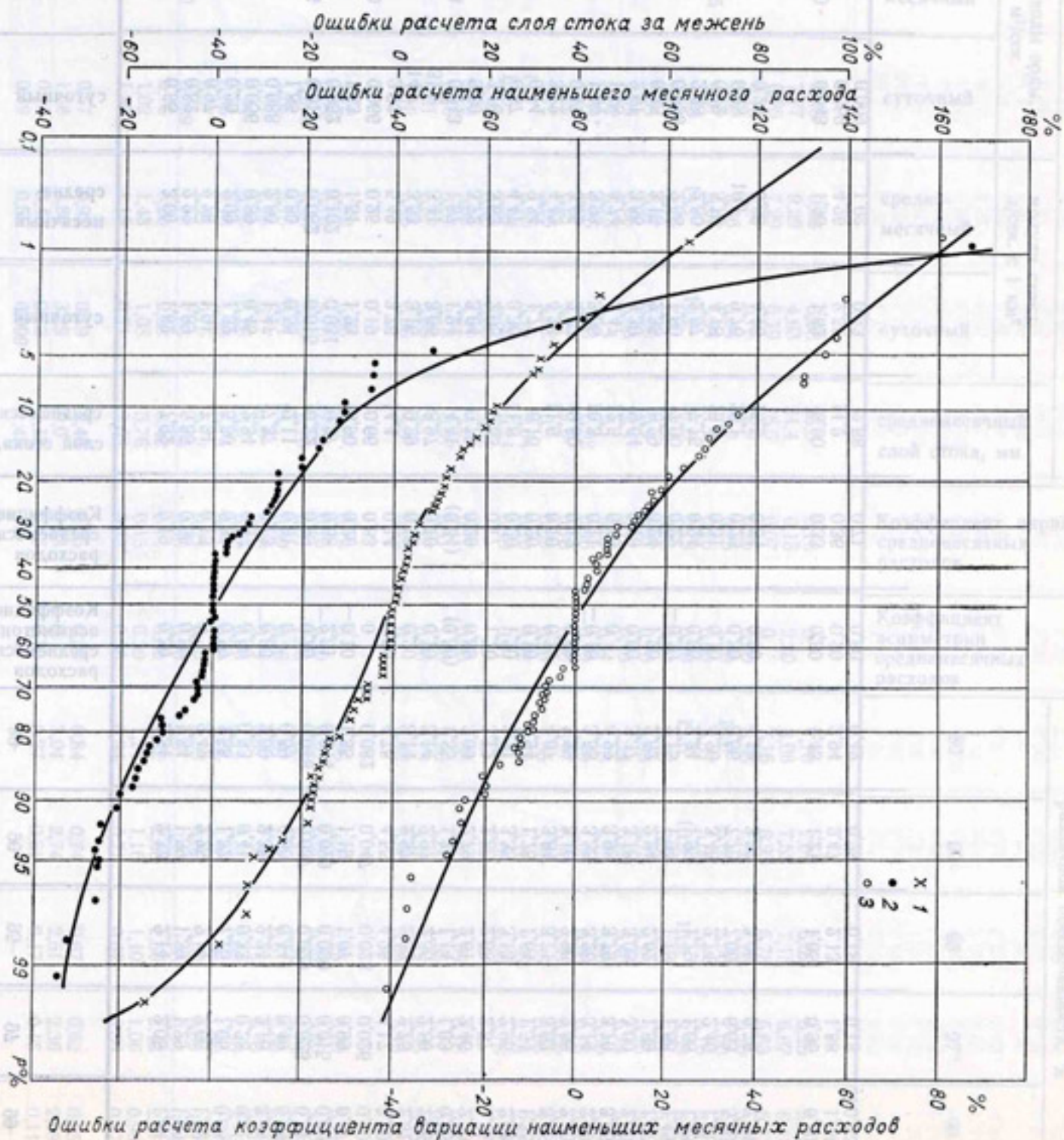
Рис. 76. Обеспеченность относительных ошибок расчета слоя стока за межень (1), минимального месячного слоя (2) и коэффициентов вариации минимального месячного стока (3).
