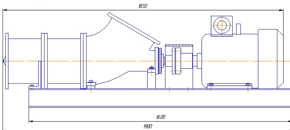
Рис. 6 - Насосный агрегат ОГ8-25х2.
