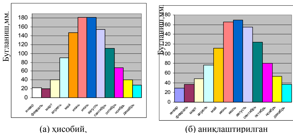
Расм. 1-Тўдакўл сув омбори юзасидаги ойлик буғланиш диаграммаси.
