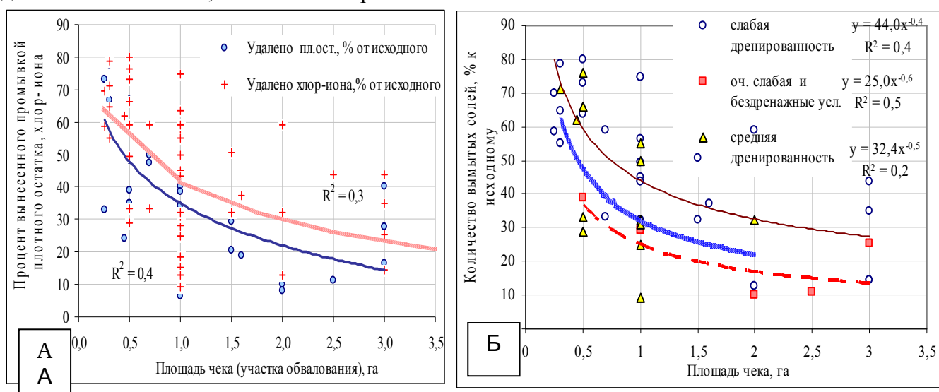
Рис. 1 - Влияние размеров чеков на эффективность вымыва плотного остатка и хлор-иона в производственных условиях (А - общая выборка, Б - для разной степени дренированности) по данным наблюдений Р. Кошекова
