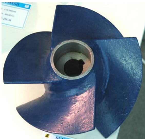
Рис. 4 - Рабочее колесо насоса ОГ8-25.
