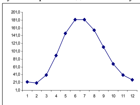
Расм. 2-Тўдакўл сув омбори юзасидаги буғланишни аниқлаштирилган ҳисобий эгри чизиги.
