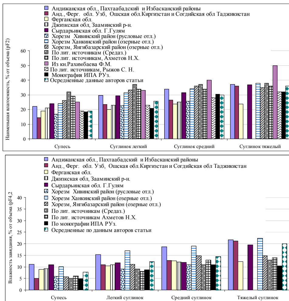
Рис. 5 - Иллюстрация расхождений значений НВ и ВЗ для почв одинаковых по мех. составу при разном происхождении и средние показатели, приведенные в отечественных литературных источниках [4, 7, 8, 11, 12]
