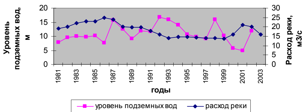
Рис.3. Среднегодовые уровни подземных вод на линии ВУ-1 и расходы реки Акдаря
