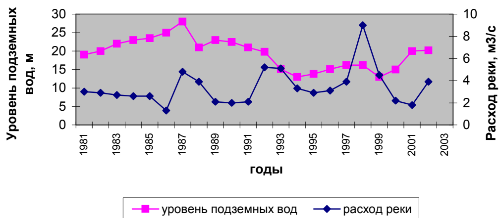
Рис.2-Среднегодовые уровни подземных вод на линии ВУ-1 и расходы реки Танхаздаря
