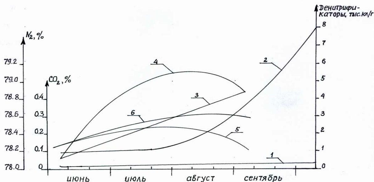
Рис. 2 - Динамика численности денитрификаторов (1, 2), концентрации молекулярного азота (3, 4), углекислого газа (5, 6) в эмитированном почвой воздухе из открытой (1, 3, 5) и мульчированной почвы (2, 4, 6).
