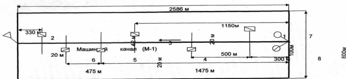
Рис. 1 - Схема севооборотного массива орошаемого машиной «Valley» с расположением почвенных разрезов: 1, 2, 3, 4, 5, 6 – почвенные разрезы; 7 - водовыпуск; 8 - насосная станция; 9 - сбросное сооружение.
