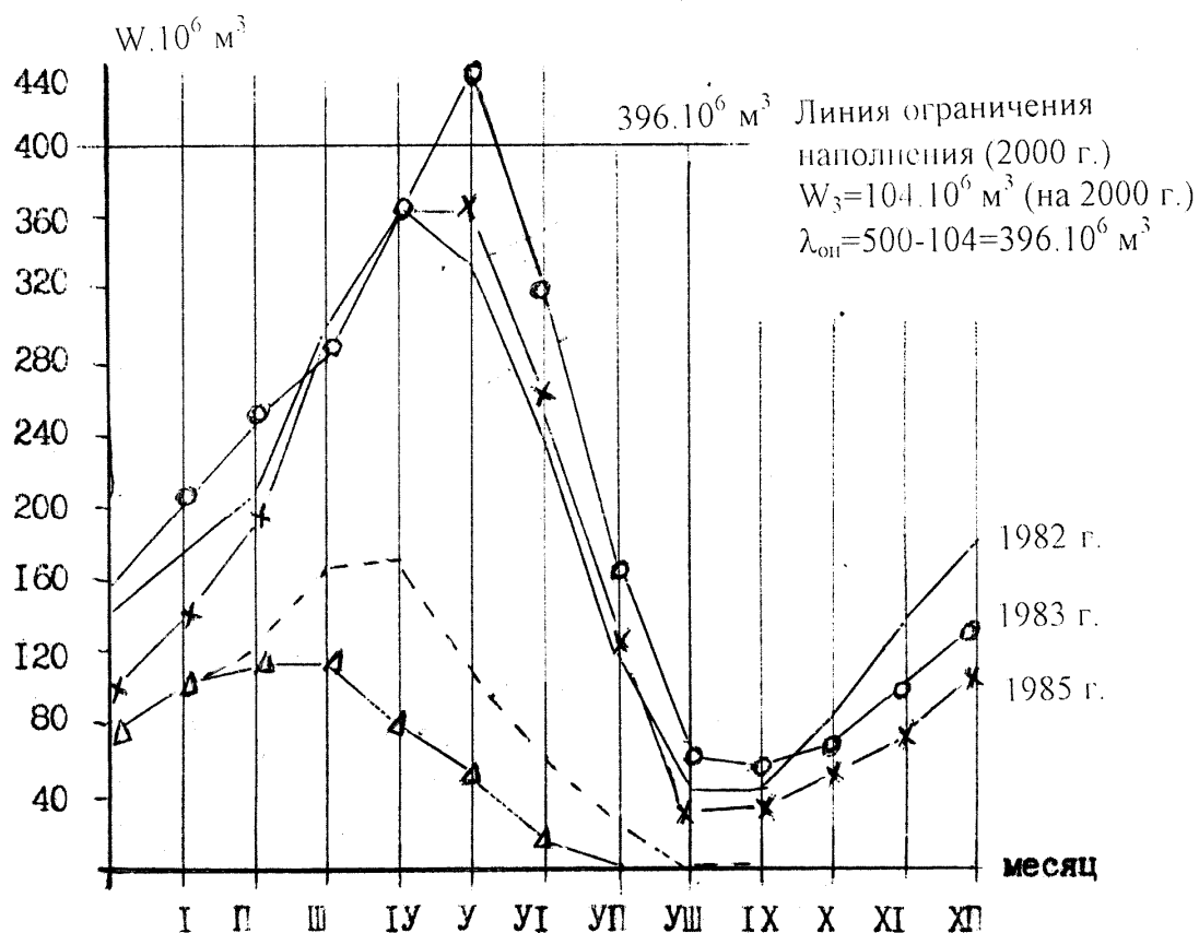
Рис. 3. Режим наполнения и сбросов Чимкурганского водохранилища для лет различной водности
