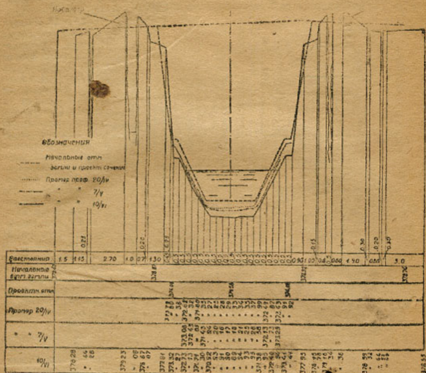
Рис. 18. Средний профиль участка Старого Дзюна.
