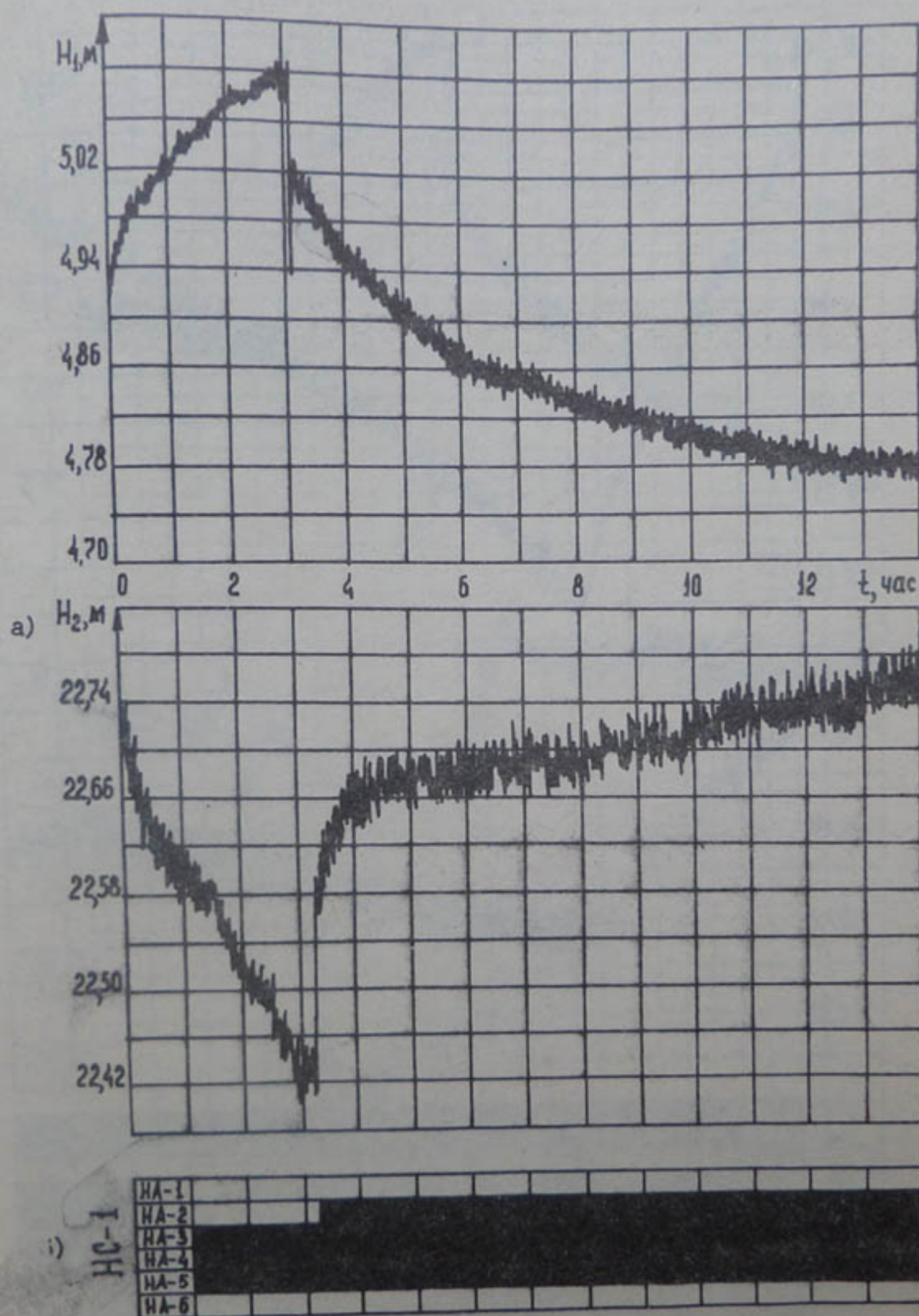
Рис. 2. Изменение режима работы НС-1 в первом эксперименте.
