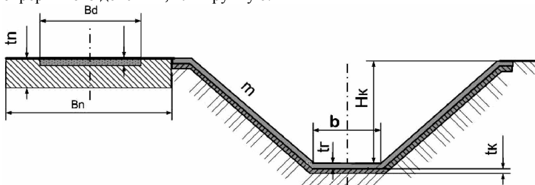
Рис. 1 - Конструкция противофильтрационного экрана из местных материалов b -ширина по дну канала; tk - толщина противофильтрационного экрана; Hк - строительная глубина канала; tg - толщина уплотненного по периметру канала грунта; Bд -ширина инспекторской дороги; m - коэффициент заложения откоса
