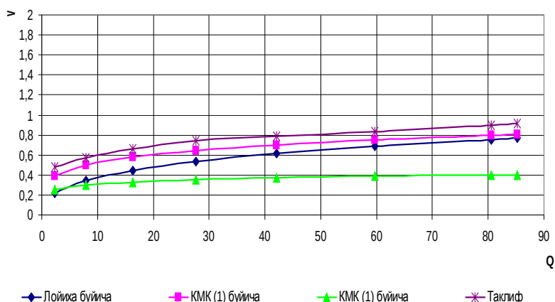
Расм 2 - Канал гидравлик элементларининг сув сарфига боғлиқ равишда узғариши графиги
