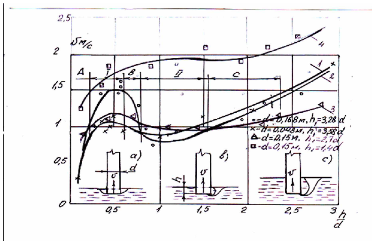
Рис. 1. График зависимости критической скорости движения жидкости во всасывающей трубе от глубины погружения входного отверстия 1, 2- по данным В.П. Чуписа для чистой воды; 3-по данным автора для чистой воды; 4-по данным автора для сегментной струенаправляющей стенки с отложениями наносов в камере.
