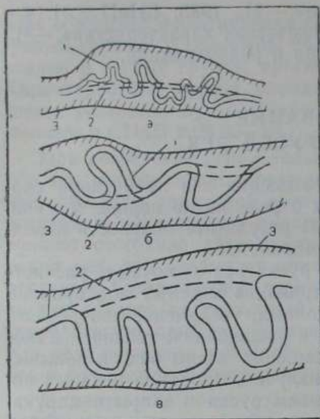
Рис. 13. Способы спрямления русел рек: а — при малых размерах сильноизвилистого русла — новое русло; б — короткие прокопы; в — решительное спрямление; 1 — естественное русло; 2 — проектируемая трасса реки (спрямление); 3 — коренной берег поймы реки
