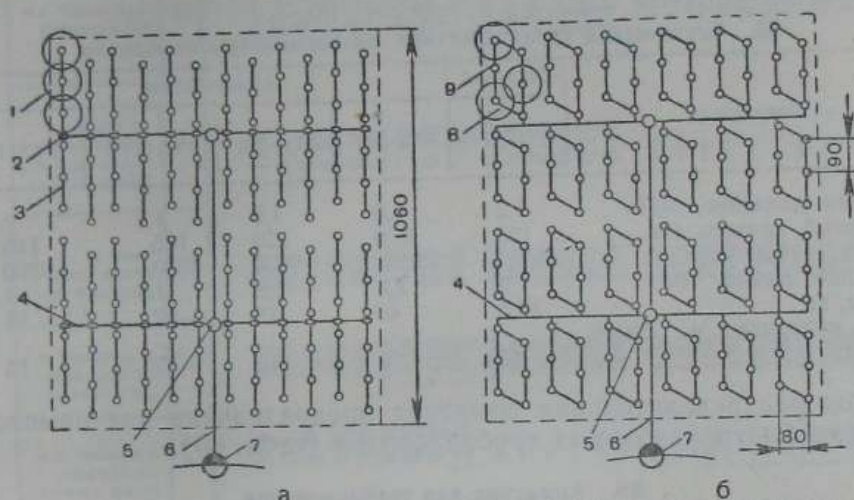
Рис. 21. Схемы автоматизированных дождевальных систем площадью 100 га: а — тупиковой сети; б — кольцевой; 1 — дождевальный аппарат ДД-30; 2 — колодец управления; 3 — поливной трубопровод тупиковый; 4 — распределительный трубопровод; 5 — распределительный колодец; 6 — магистральный трубопровод; 7 — насосная станция; 8 — дождевальный аппарат ДД-30 с гидрозатвором; 9 — поливной кольцевой трубопровод
