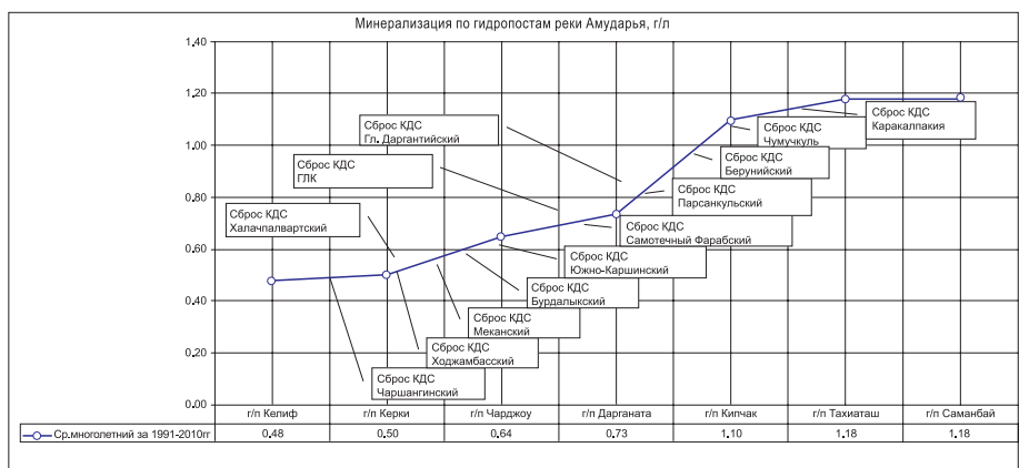
Рисунок 2.11. Рост минерализации воды по длине реки Амударьи (Качество воды в бассейнах рек Амударьи и Сырдарья. Аналитический отчёт. НИЦ МКВК, ЕЭК ООН, РЭЦ ЦА. Ташкент 2011 г.)
