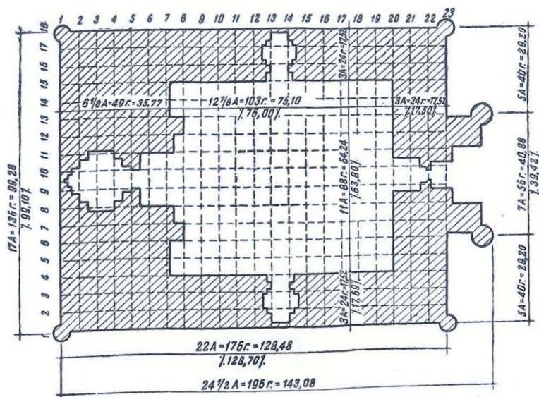
Рис. 82. Биби-ханым. Анализ построения плана всего комплекса мечети.
