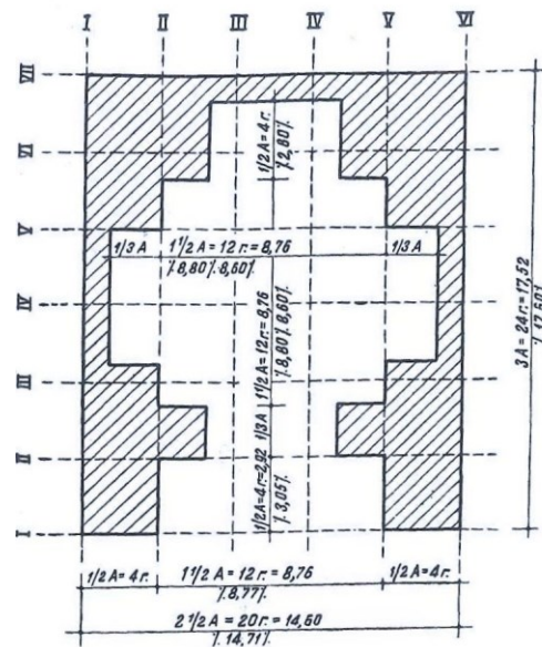
Рис. 81. Биби-ханым. Анализ построения плана малых мечетей комплекса.
