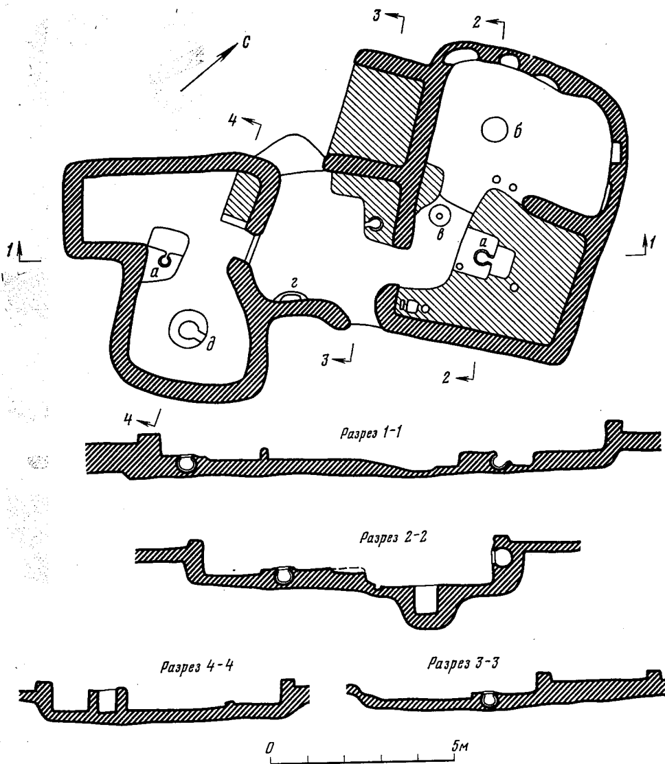
Рис. 4. Дом № 2 в Куня-Узском поселении середины XIV в.
