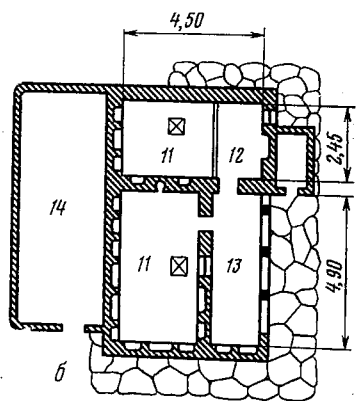
Рис. 2. План дома семьи Сафаровых в кишлаке Хишертуб. Ягноб, 1971 г.
