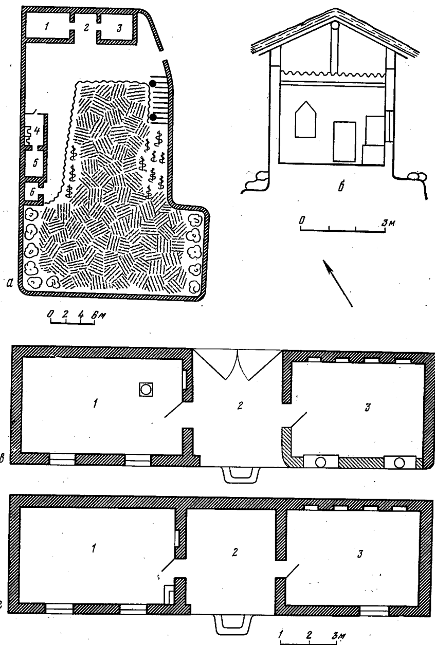
Рис. 3. План усадьбы и жилых домов, построенных в кishлаке Туткавул
