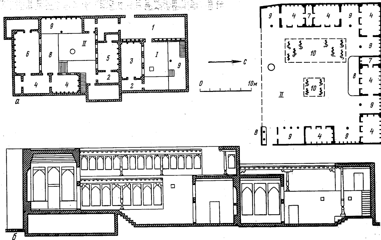
Рис. 1. Периметральная застройка двора
