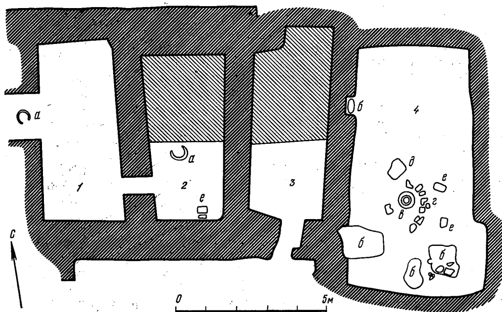
Рис. 2. Дом № 41 в поселении середины XIV в. близ Ак-калы а — очаги, б — ямы, в — тандыр, з — обломки жерновов, д — пахсовое возвышение, е — кирпичи
